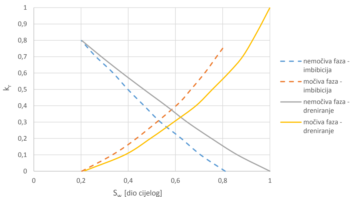
Slika 3-1. Krivulje relativnih propusnosti za močivu i nemočivu fazu, ovisno o smjeru zasićenja (modificirano od Vulin, 2016)
