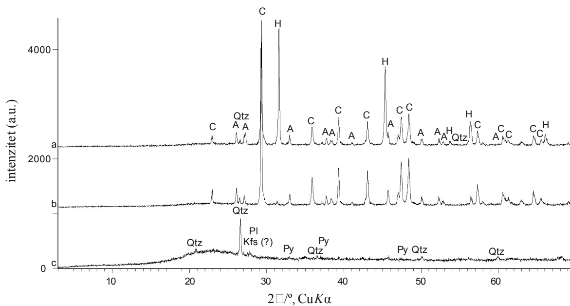
Slika 3-13. Rendgenska difrakcijska slika praha površinskog sedimenta jezgre 24-26 cm; a- originalni uzorak, b-uzorak nakon uklanjanja halita, c-uzorak nakon otapanja karbonata u acetatnoj kiselini.
