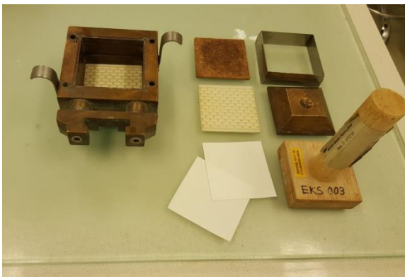
Slika 3-21. (a) Potrebni pribor prilikom ugradnje, (b) Uzorak ugrađen u prsten
