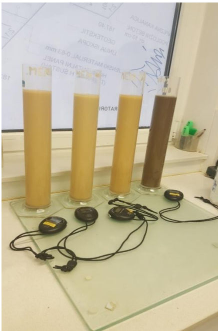
Slika 3-10. Postupak areometriranja
