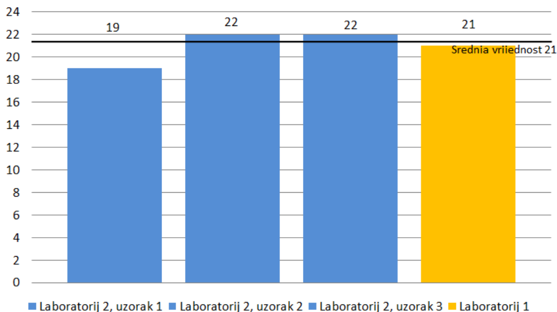
Slika 3-7. Vrijednosti rezultata indeksa plastičnosti
