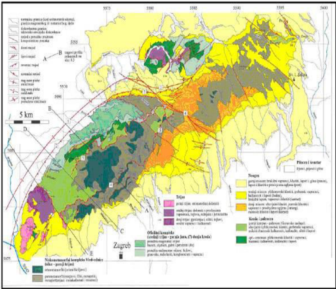
Slika 4: Geološka karta Medvednice (preuzeto: Šikić, 1995)
