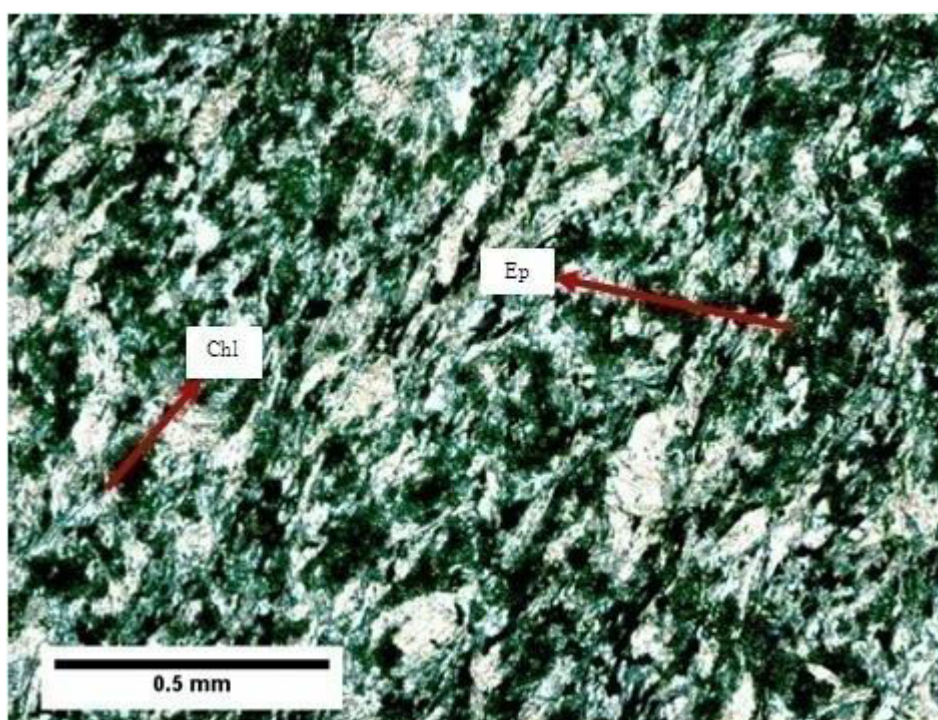
Slika 65: Mikroskopski preparat 5143, bez analizatorom
