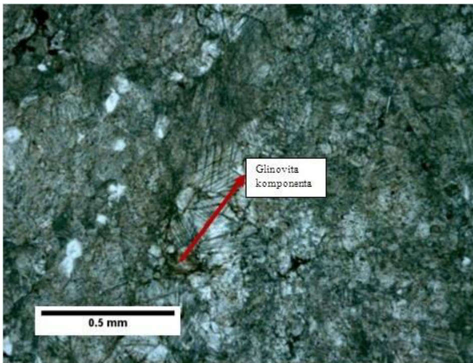
Slika 82: Mikroskopski preparat 5144, bez analizatora
