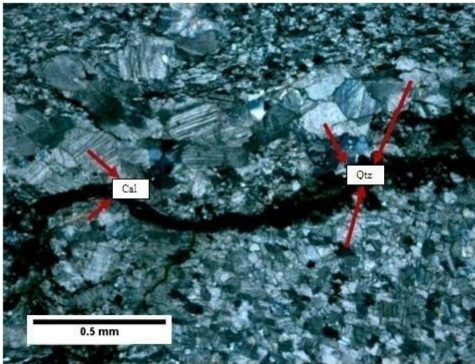
Slika 87: Mikroskopski preparat 5142, s analizatorom
