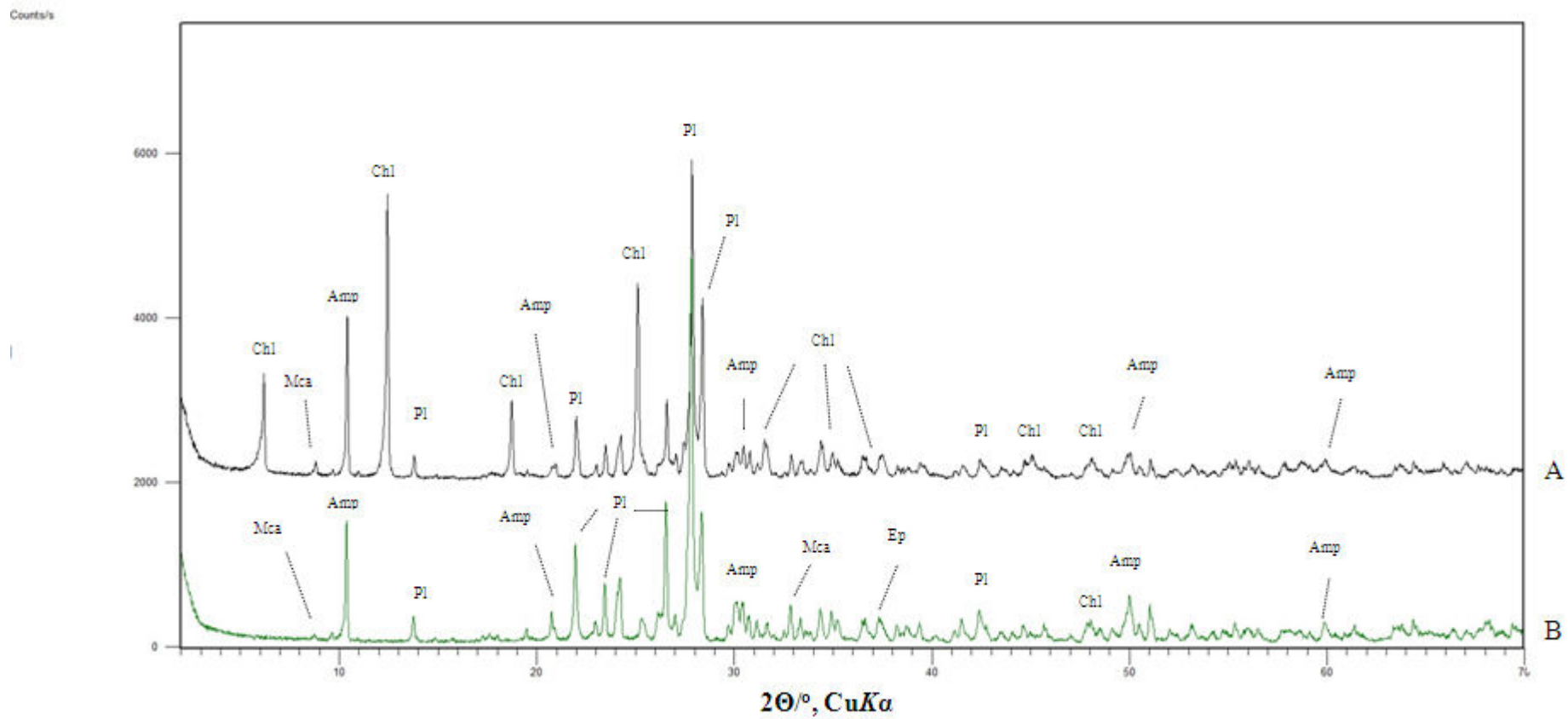
Prilog 9. Difrakcijske slike uzorka 5121 (LUG 1)
