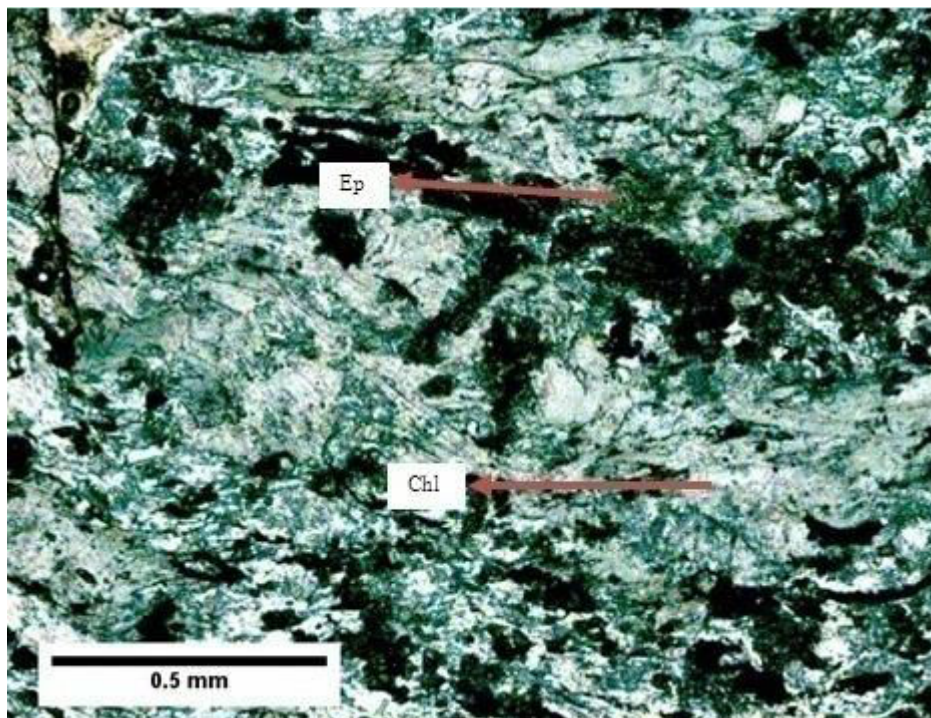
Slika 57: Mikroskopski preparat 5140, bez analizatora
