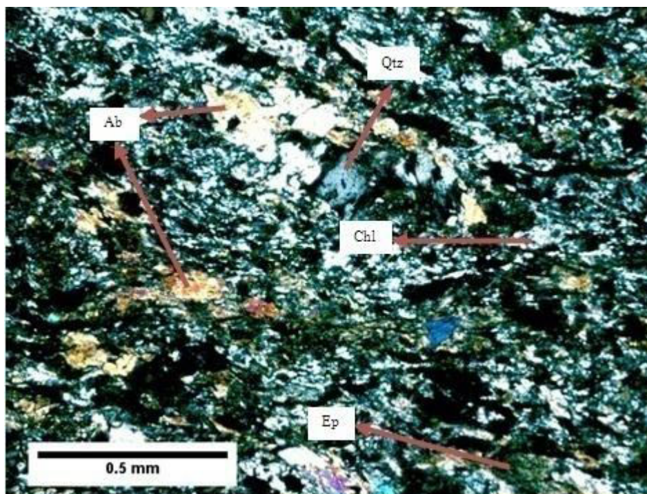
Slika 60: Mikroskopski preparat 5140, sa analizatorom
