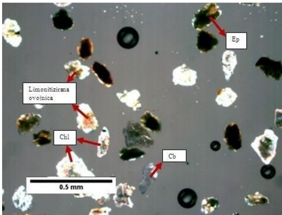
Slika 54: Mikroskopski preparat 5135, s analizatorom
