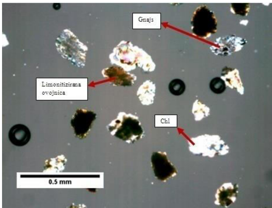
Slika 42: Mikroskopski preparat 5134, s analizatorom
