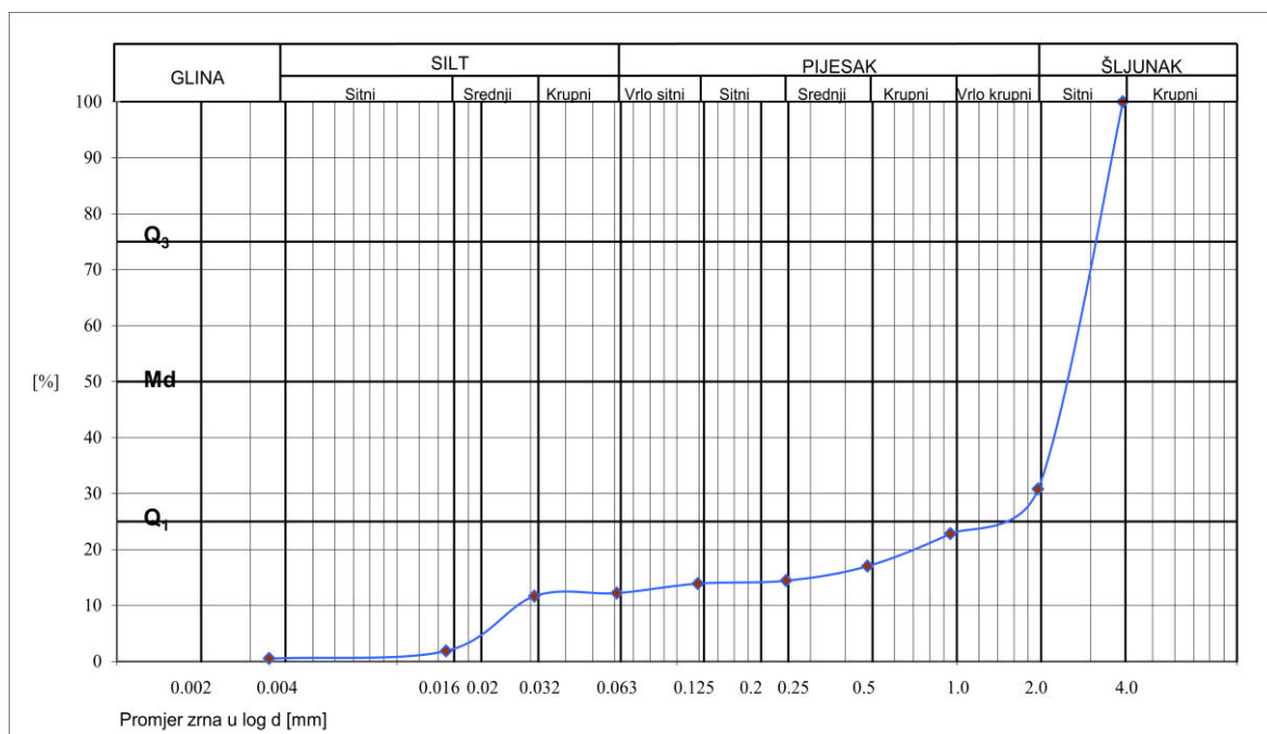
Slika 31: Granulometrijska krivulja uzorka točke LUG 1
