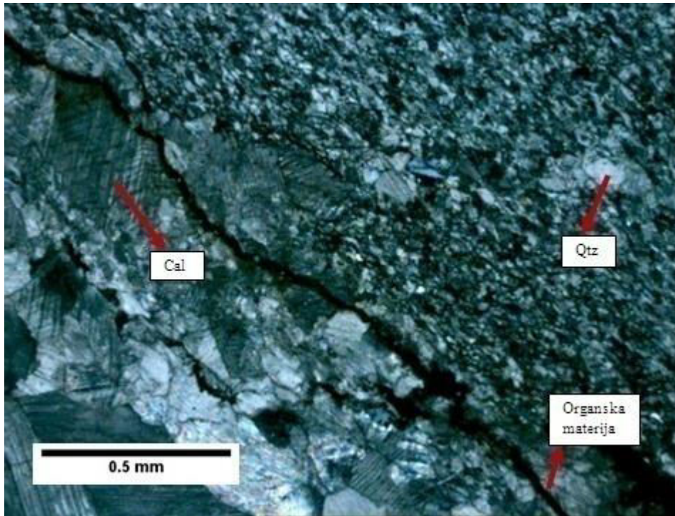
Slika 89: Mikroskopski preparat 5142, s analizatorom
