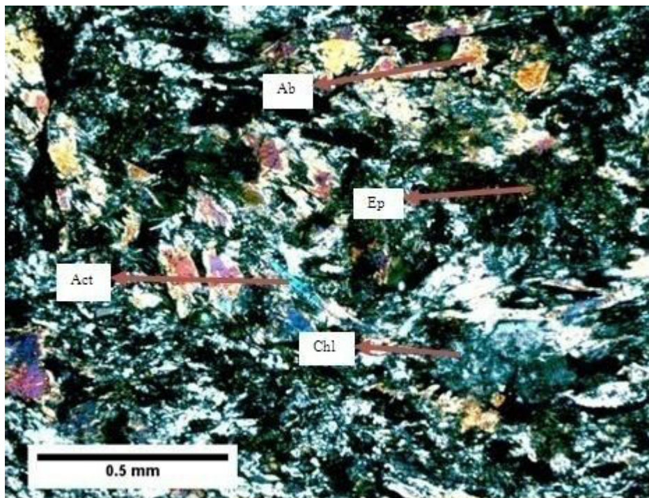
Slika 58: Mikroskopski preparat 5140, s analizatorom
