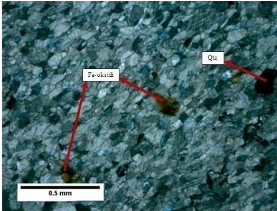
Slika 77: Mikroskopski preparat 5141, sa analizatorom
