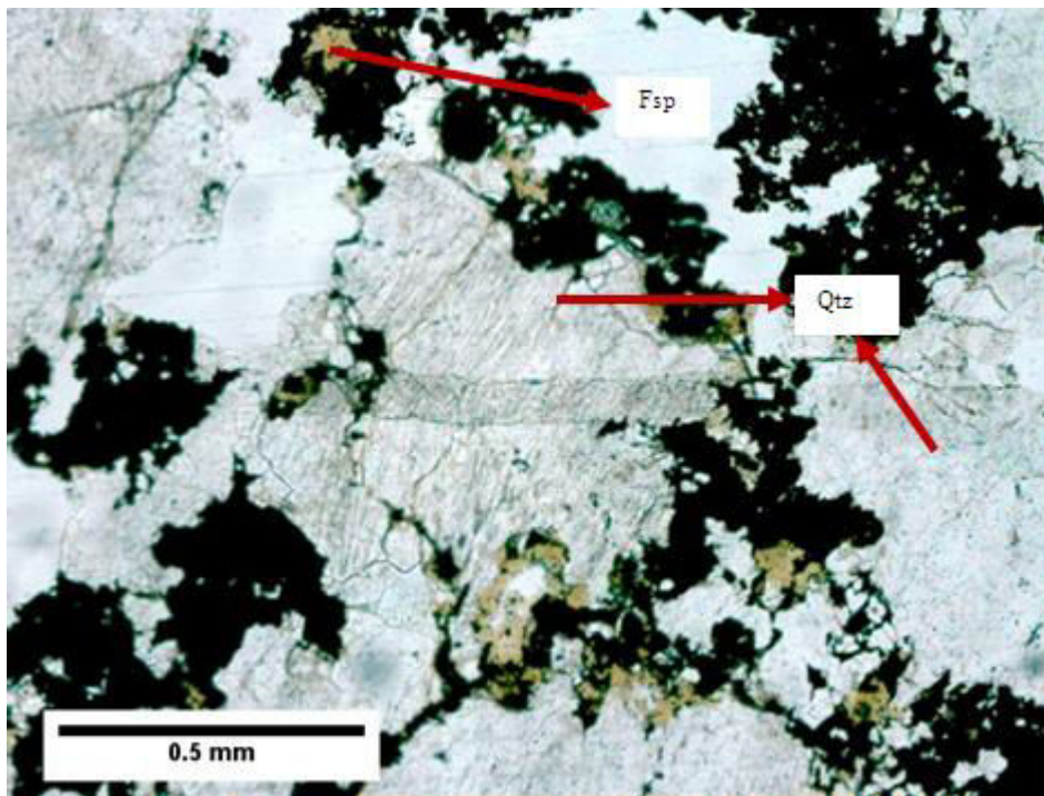
Slika 71: Mikroskopski preparat 5145, bez analizatora
