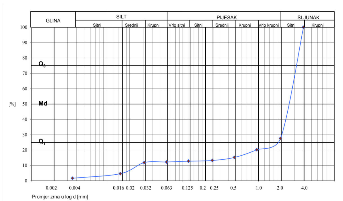
Slika 15: Granulometrijska krivulja uzorka točke Izvor 1
