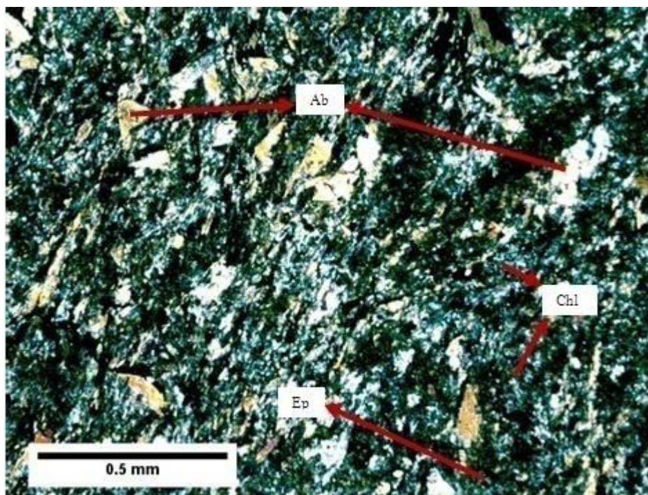
Slika 64: Mikroskopski preparat 5143, s analizatorom
