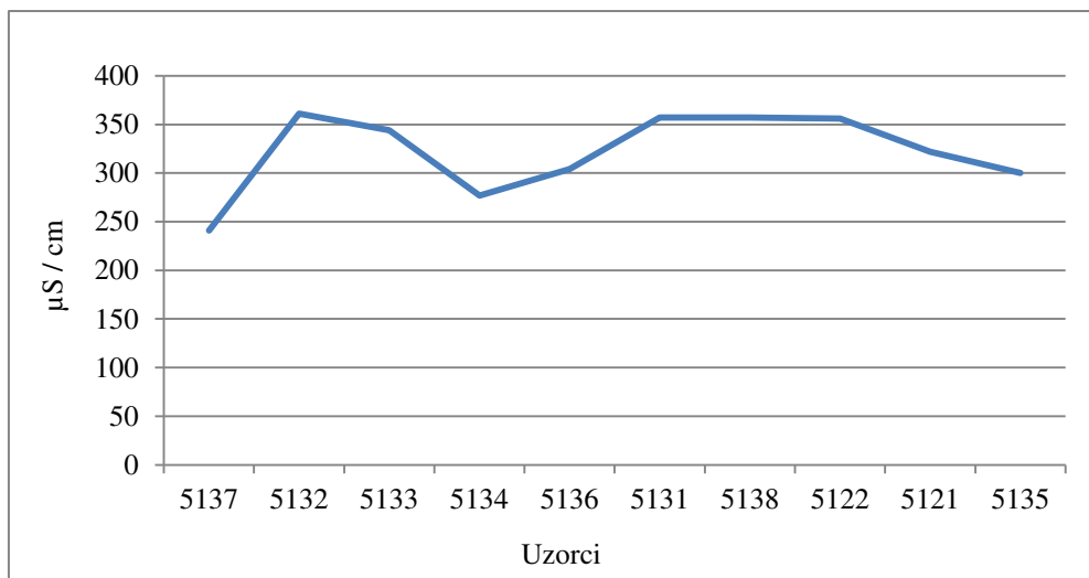
Slika 11: Električna vodljivost vode potoka
