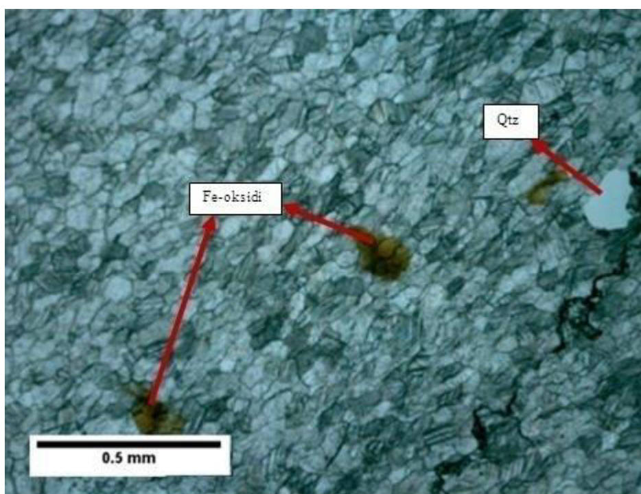
Slika 76: Mikroskopski preparat 5141, bez analizatora
