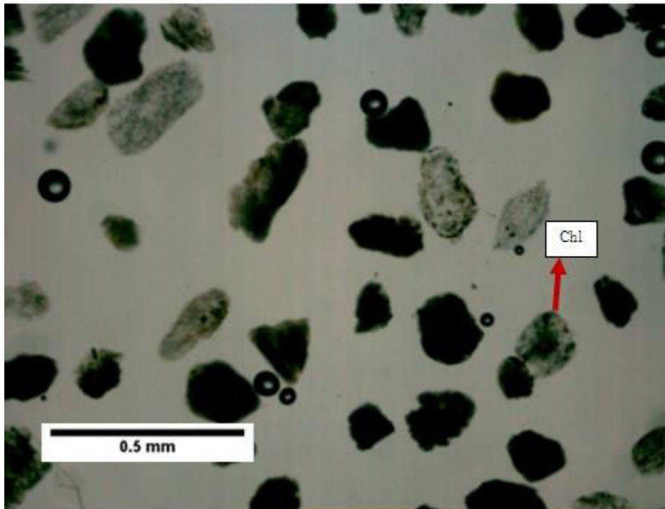
Slika 39: Mikroskopski preparat 5133, bez analizatora
