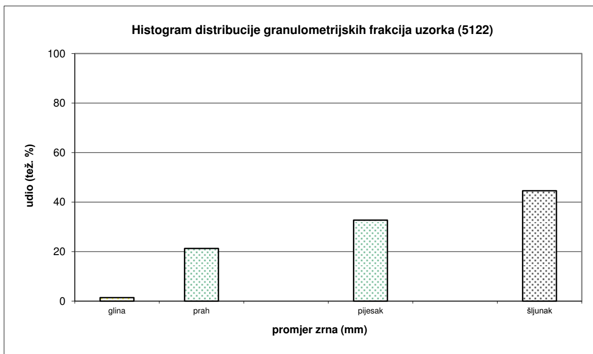
Slika 30: Histogram distribucije granulometrijskih frakcija uzorka točke LUG 2
