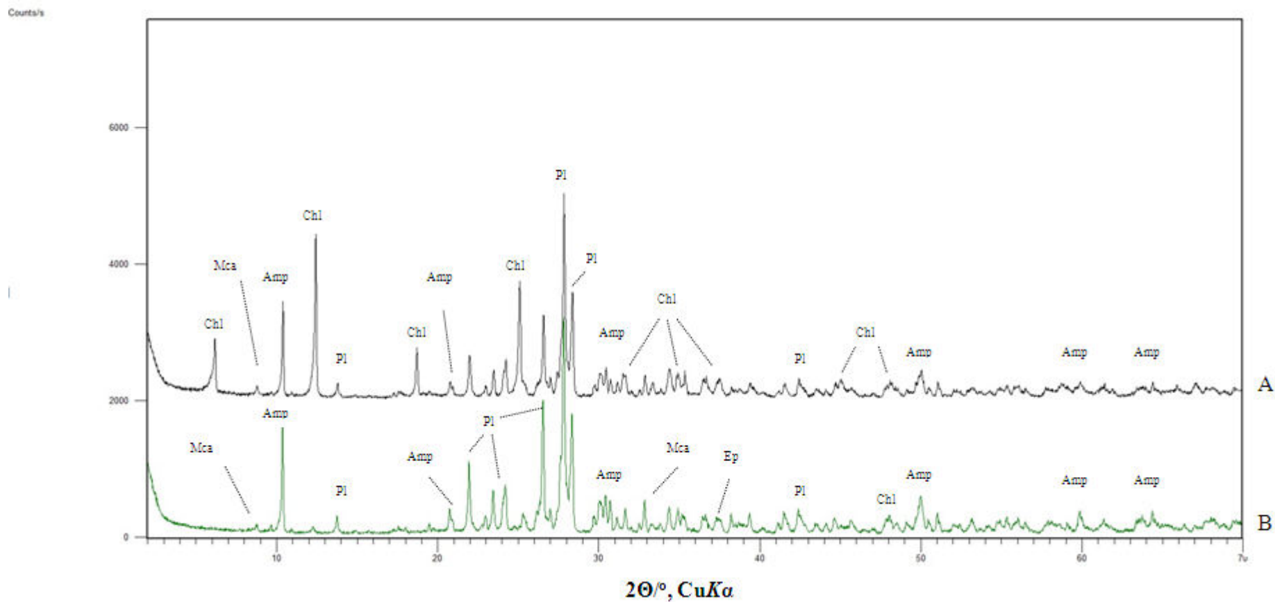
Prilog 8. Difrakcijske slike uzorka 5122 (LUG 2)
