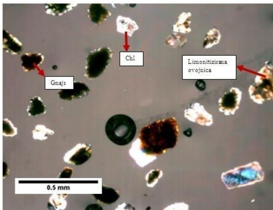
Slika 36: Mikroskopski preparat 5137, sa analizatorom
