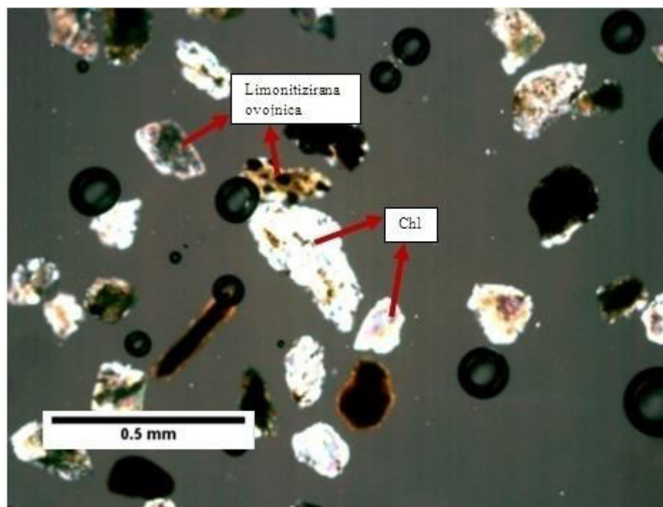
Slika 44: Mikroskopski preparat 5136, s analizatorom
