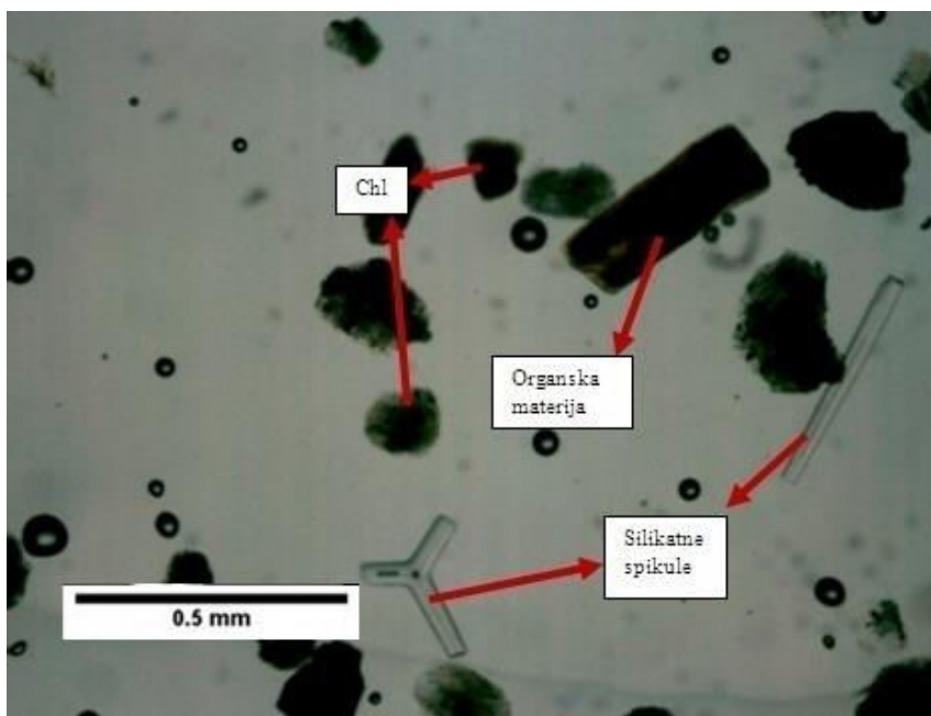
Slika 47: Mikroskopski preparat 5138, bez analizatora
