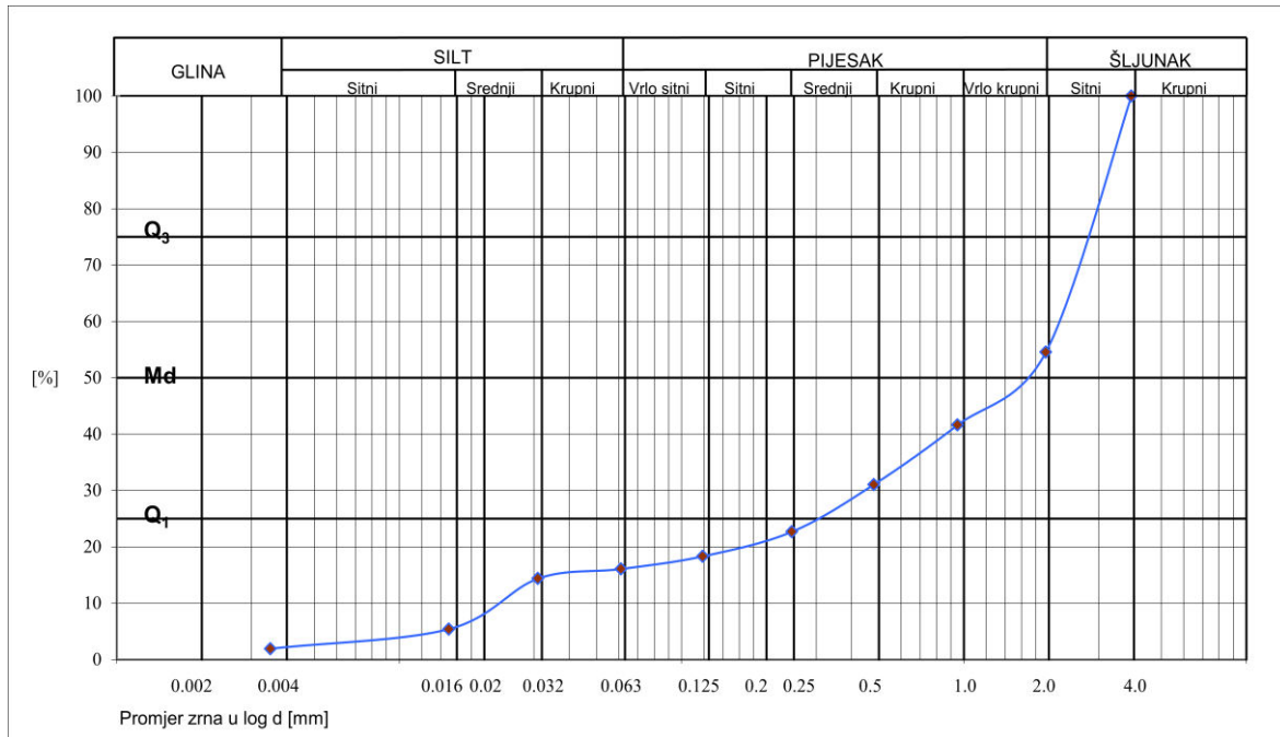
Slika 21: Granulometrijska krivulja uzorka točke T.P.M.
