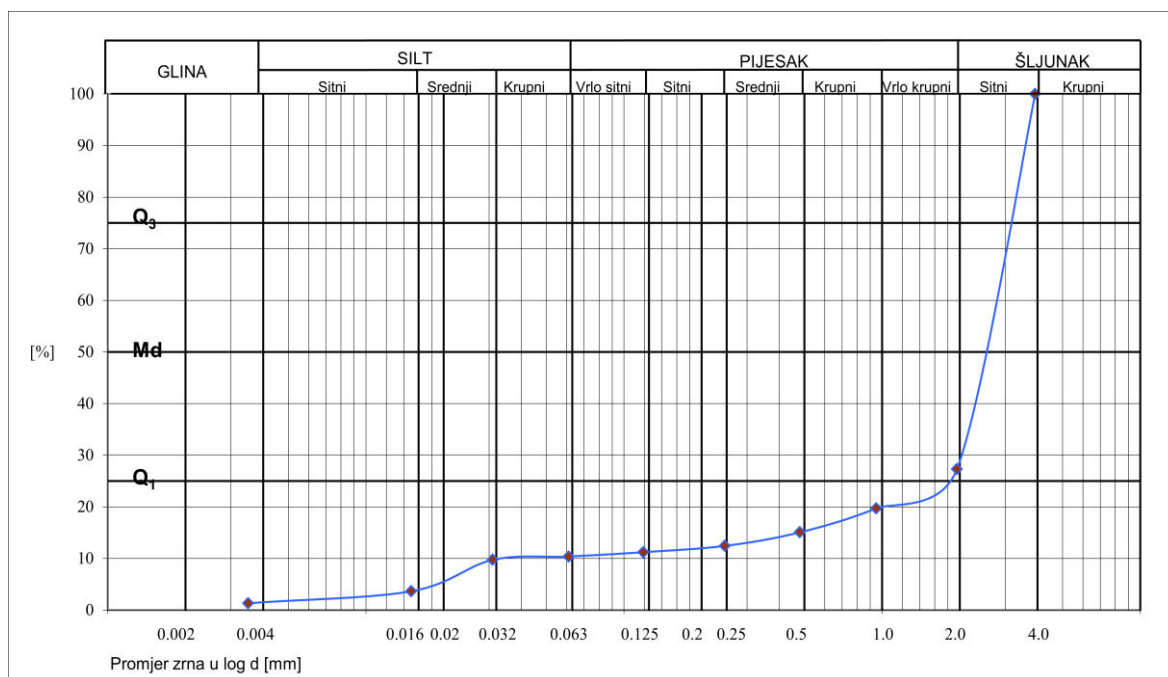
Slika 19: Granulometrijska krivulja uzorka točke Spoj oba izvora
