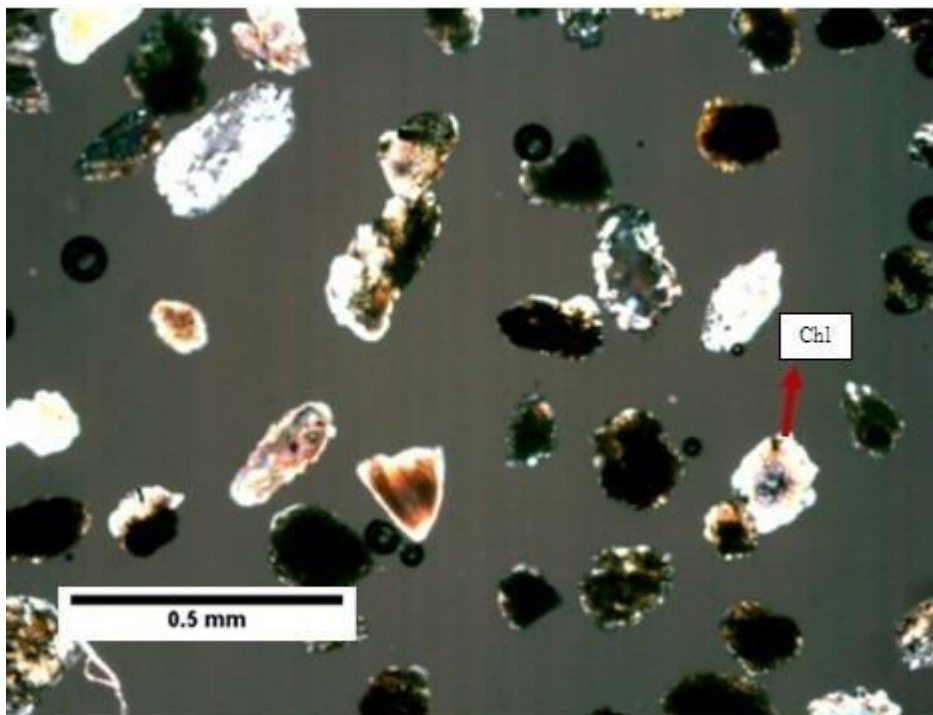
Slika 40: Mikroskopski preparat 5133, sa analizatorom
