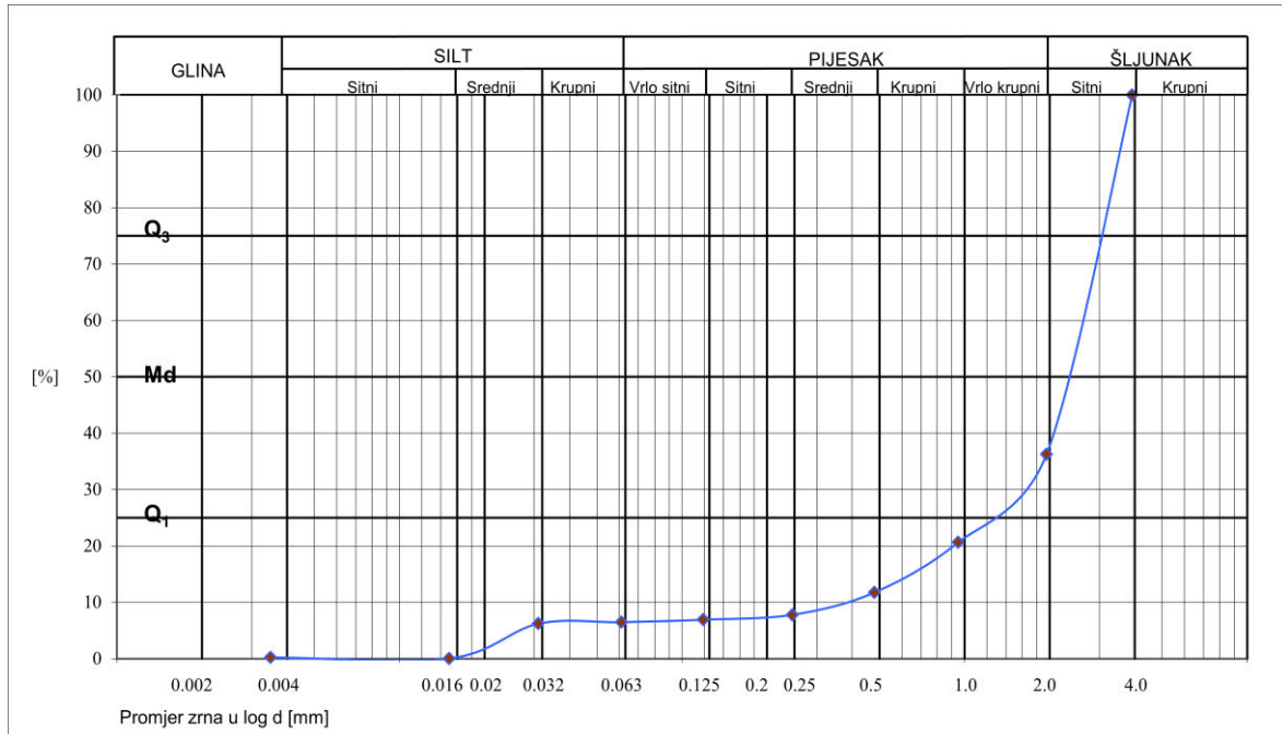
Slika 25: Granulometrijska krivulja uzorka točke S.D.D.
