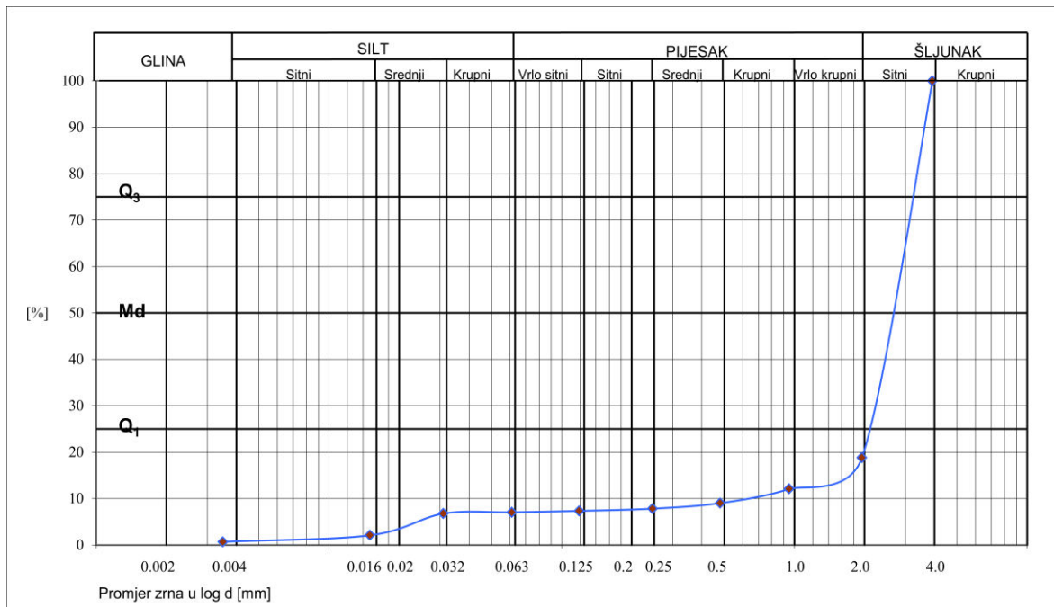
Slika 23: Granulometrijska krivulja uzorka točke T.N.M.
