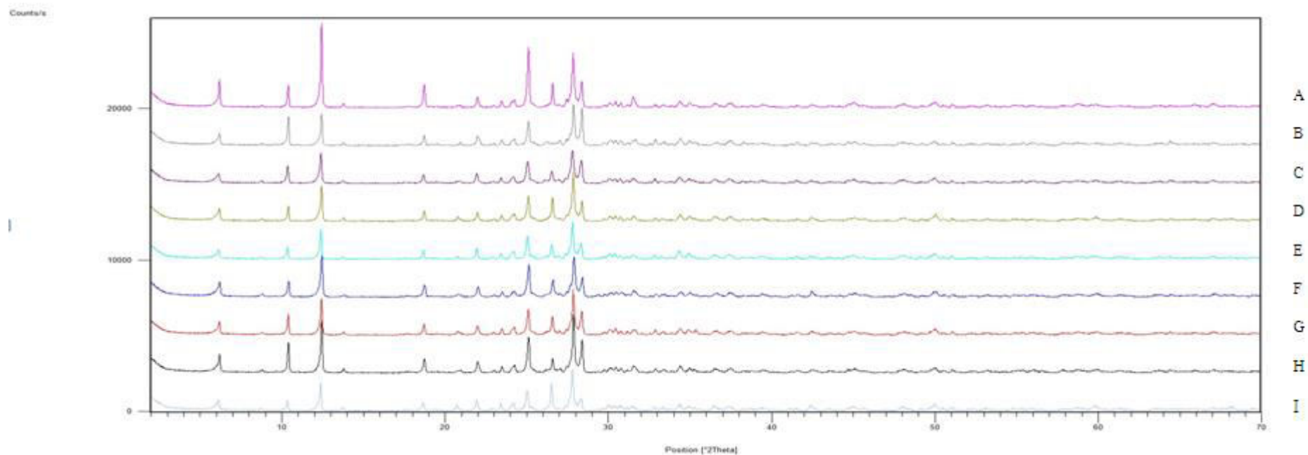
Prilog 11. Usporedba difrakcijskih slika uzoraka poredanih od izvora do ušća istraživanog potoka (bez uzorka 5138)
