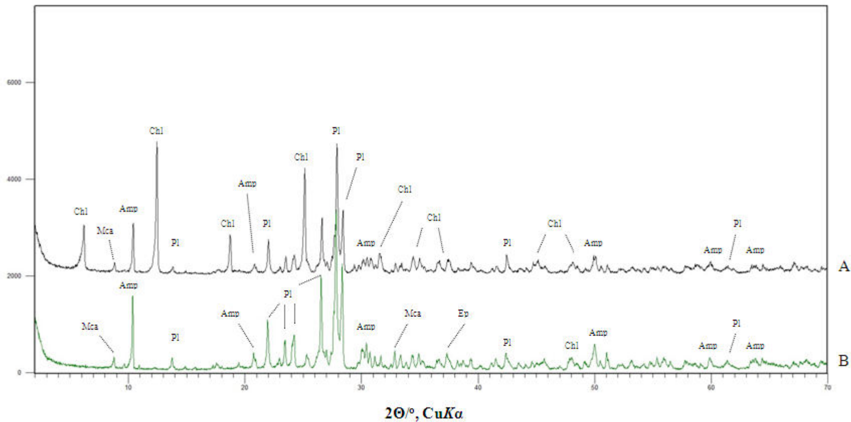
Prilog 6. Difrakcijske slike uzorka 5131 (S. D. D.)
