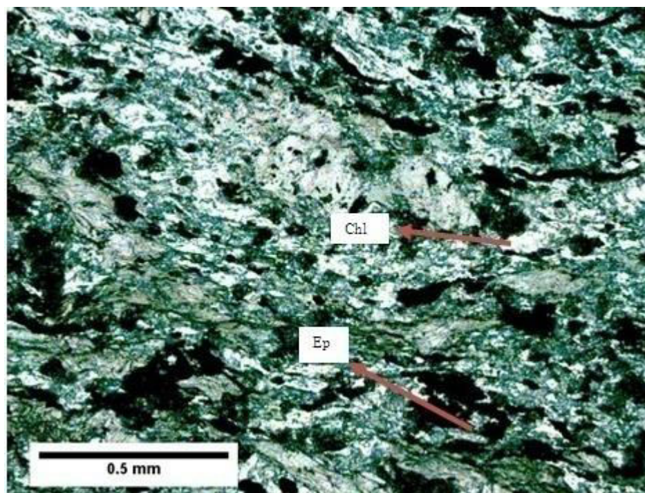
Slika 59: Mikroskopski preparat 5140, sa analizatorom
