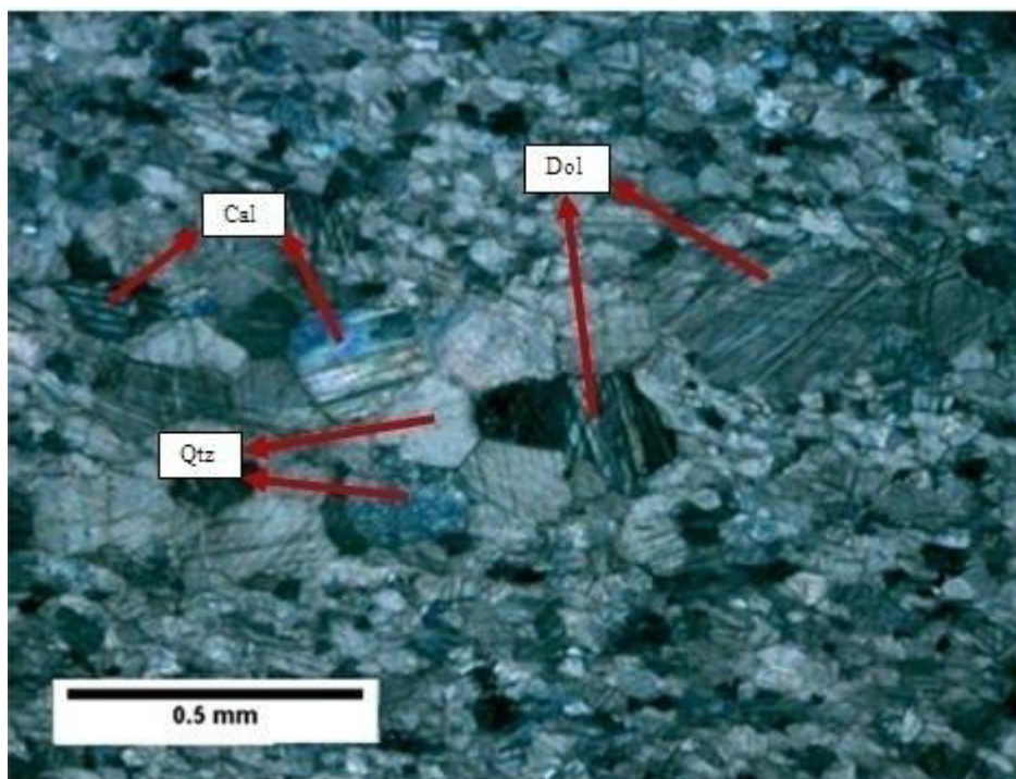
Slika 75: Mikroskopski preparat 5141, s analizatorom
