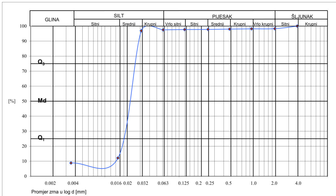
Slika 27: Granulometrijska krivulja uzorka točke S.D.D. 2
