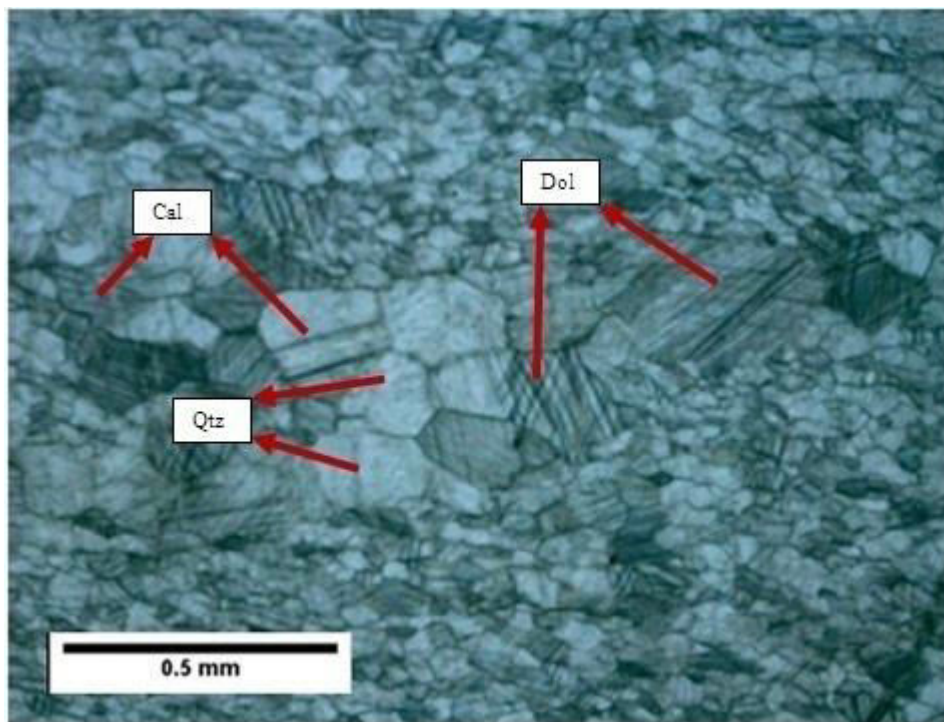
Slika 74: Mikroskopski preparat 5141, bez analizatora
