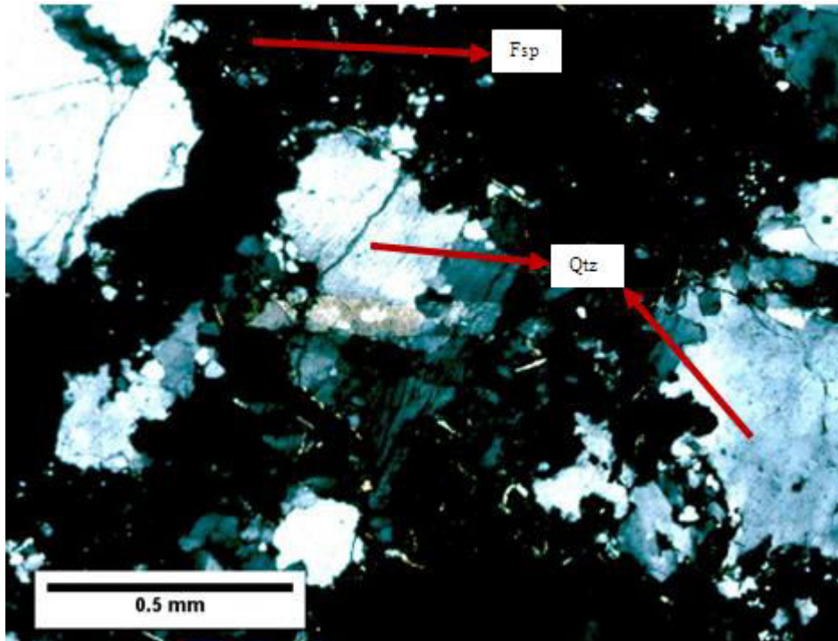
Slika 72: Mikroskopski preparat 5145, s analizatorom
