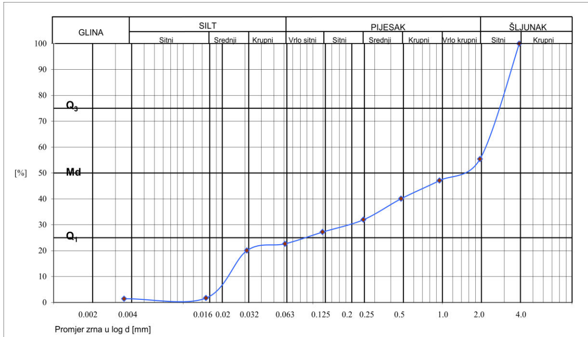
Slika 29: Granulometrijska krivulja uzorka točke LUG 2
