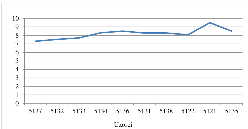
Slika 12: pH vrijednost vode potoka
