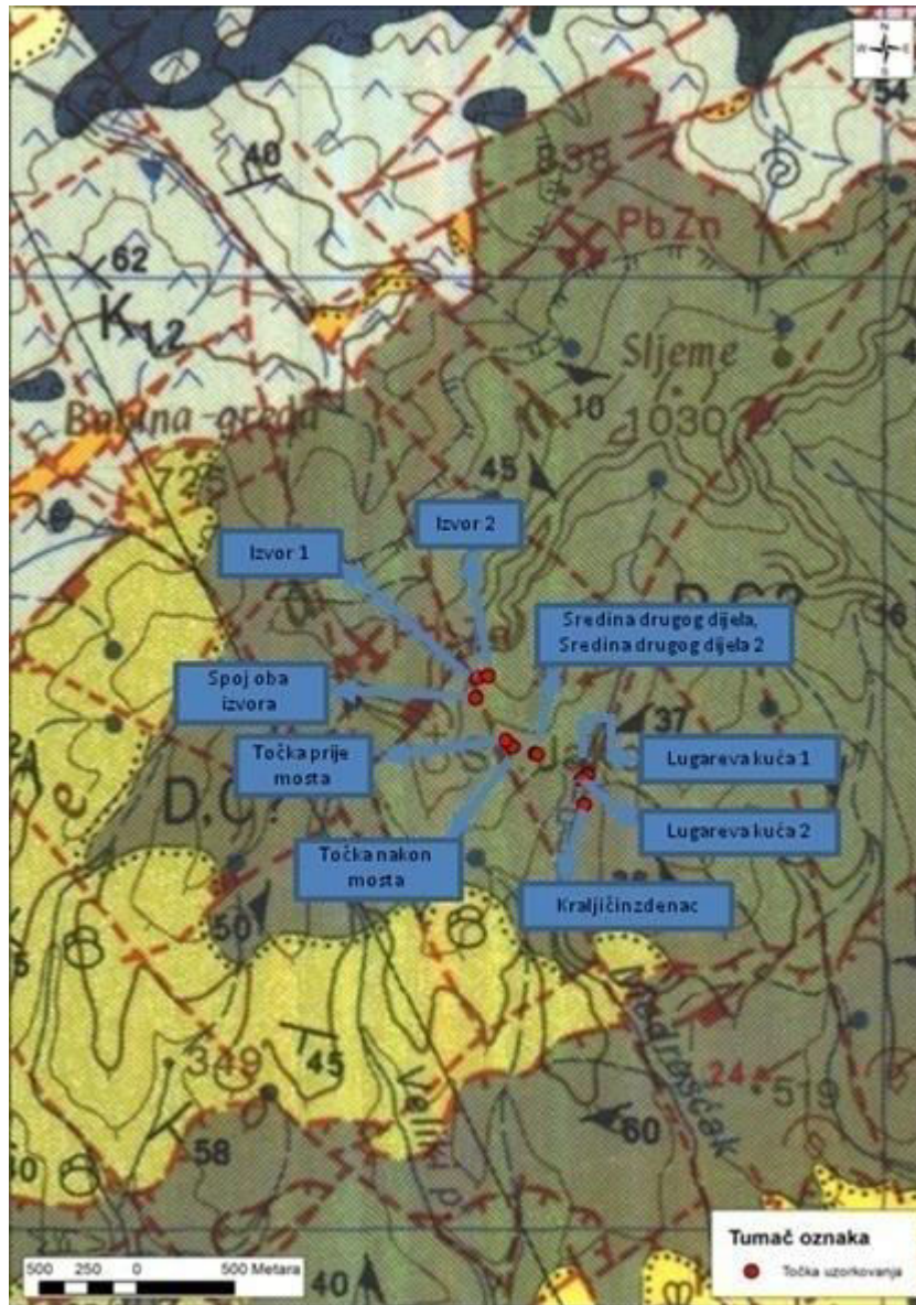
Slika 5: Prikaz točki uzorkovanja na geološkoj karti Medvednice ( modificirano prema: Šikić et al., 1977)
