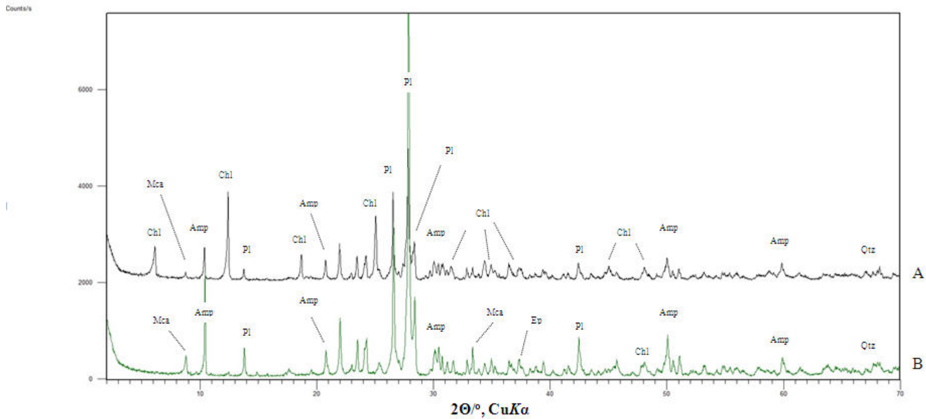
Prilog 10. Difrakcijske slike uzorka 5135 (K. Z.)
