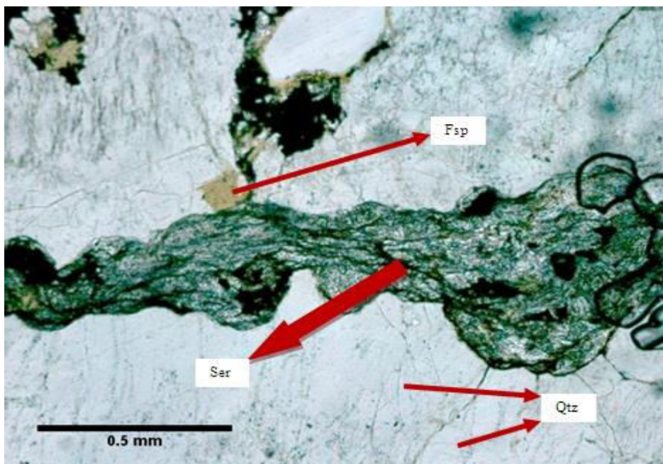
Slika 69: Mikroskopski preparat 5145, bez analizatora
