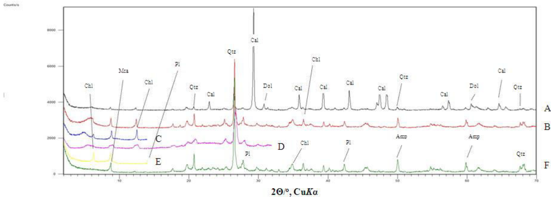
Prilog 7. Difrakcijske slike uzorka 5138 (S. D. D. 2)
