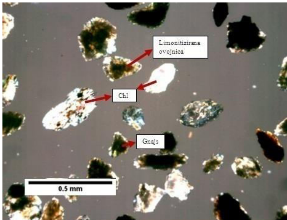
Slika 50: Mikroskopski preparat 5122, s analizatorom
