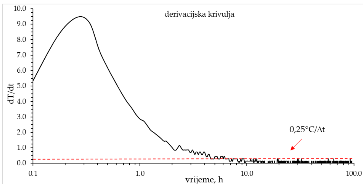
Slika 5-4. Prikaz tipičnog modela derivacijske krivulje i odabranog prijelaza iz neustaljenog u poluustaljeni period širenja toplinskog toka
