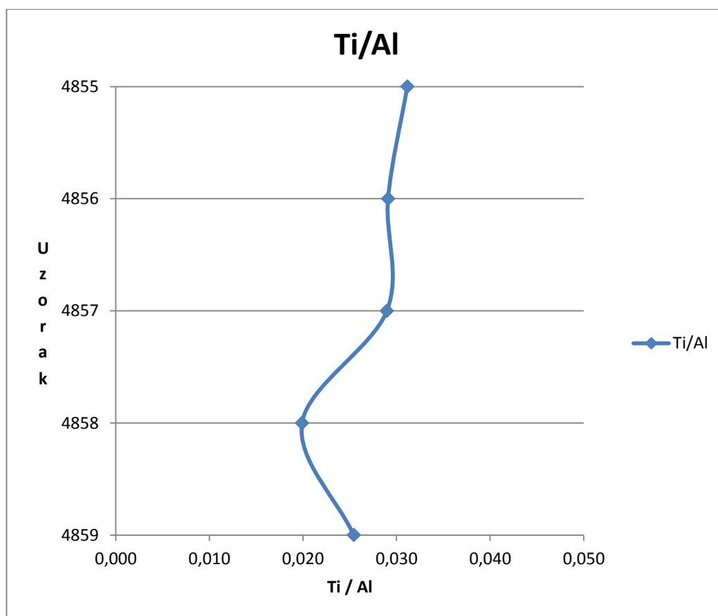
Slika 5.6. Omjer Ti/Al
