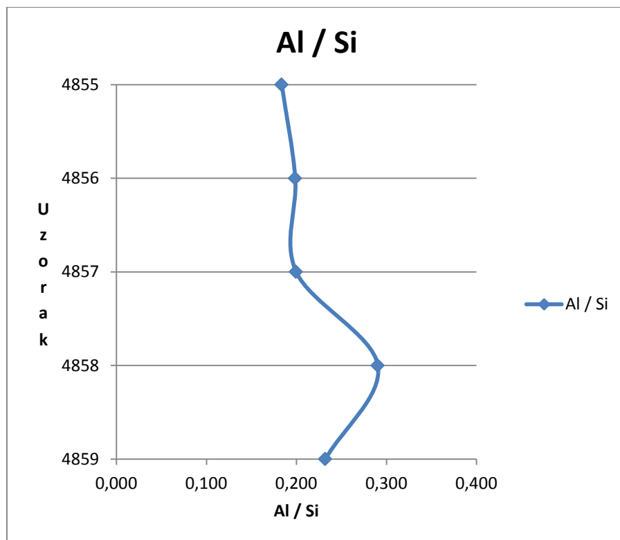
Slika 5.3. Omjer Al/Si
