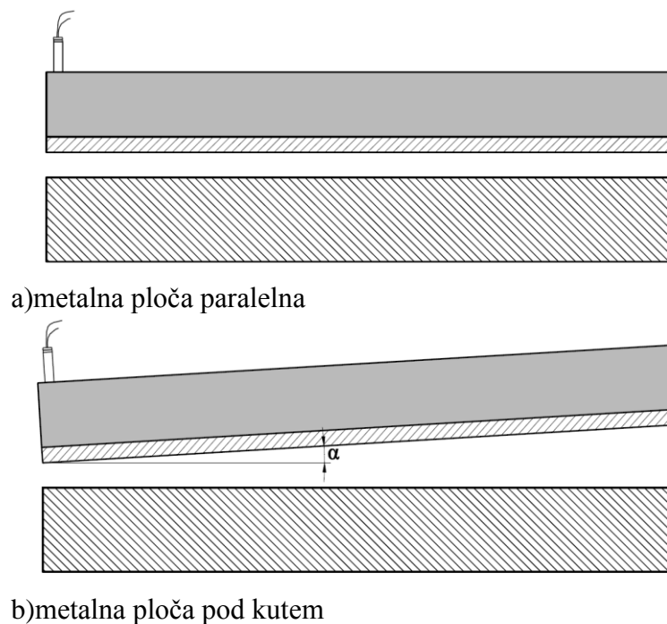
Slika 3-2. Konfiguracije koje se koriste za zavarivanje
