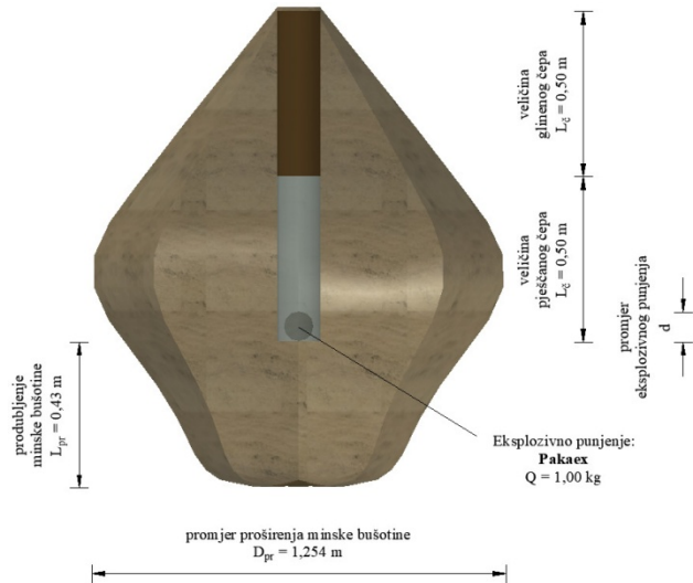
Slika 11.2 3D model nastalog proširenja minske bušotine MB 1, AutoCad Civil 3D
