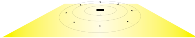
Slika 17: Kasni radijalni protok u ležištu s horizontalnom bušotinom (Houze et al., 2012)
