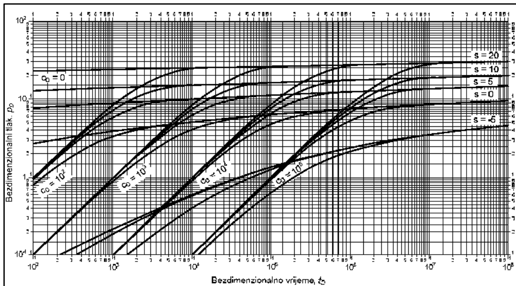
Slika 9: Bezdimezionalni tlak za bušotinu u neograničenom ležištu, s uključenim efektom skladištenja, C_D , i skin faktorom, s (Agarwal et al., 1970)
