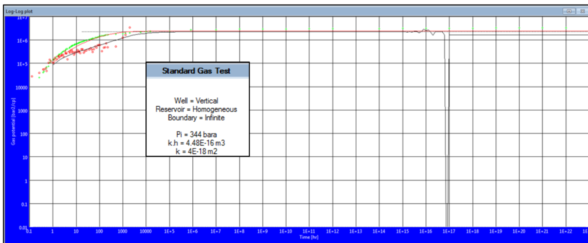
Slika 99: Log-log dijagram i rezultati analize testa porasta tlaka u programu Saphir, ležište Perth Basin
