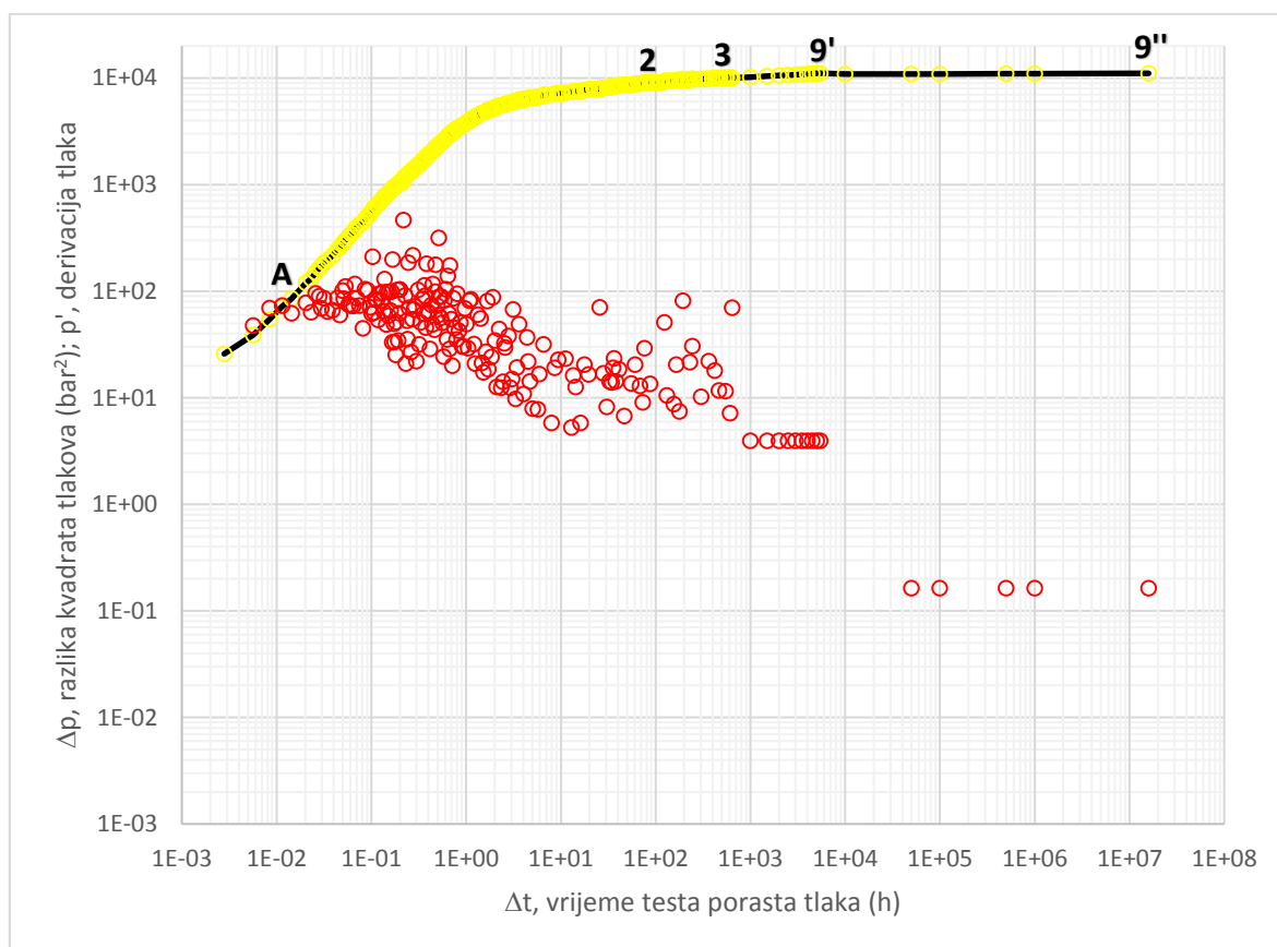
Slika 82: Derivacija krivulje testa porasta tlaka do točke 9"
