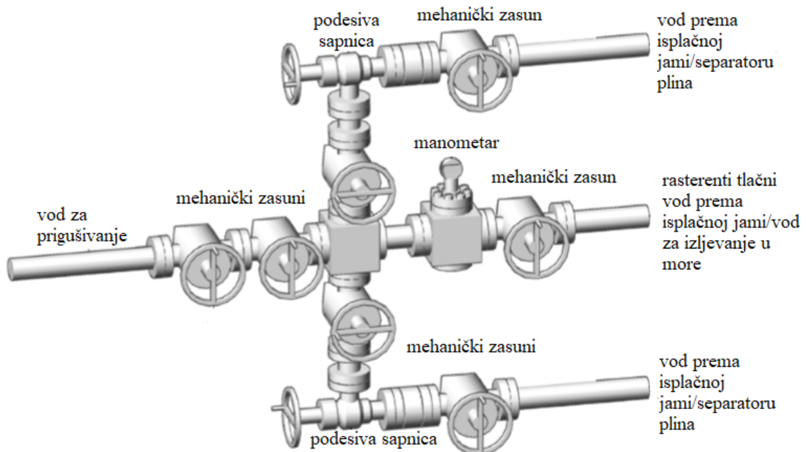
Slika 4-1. Konfiguracija razdjelnika podesive sapnice za radni tlak od 13,8/20,7 MPa (2 000/3 000) psi (API Standard 53, 2012)
