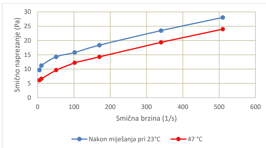
Slika 4-8. Dijagram smičnih napreznja razdjelnice za cementaciju kolone zaštitnih cijevi vanjskog promjera 13 3/8"
