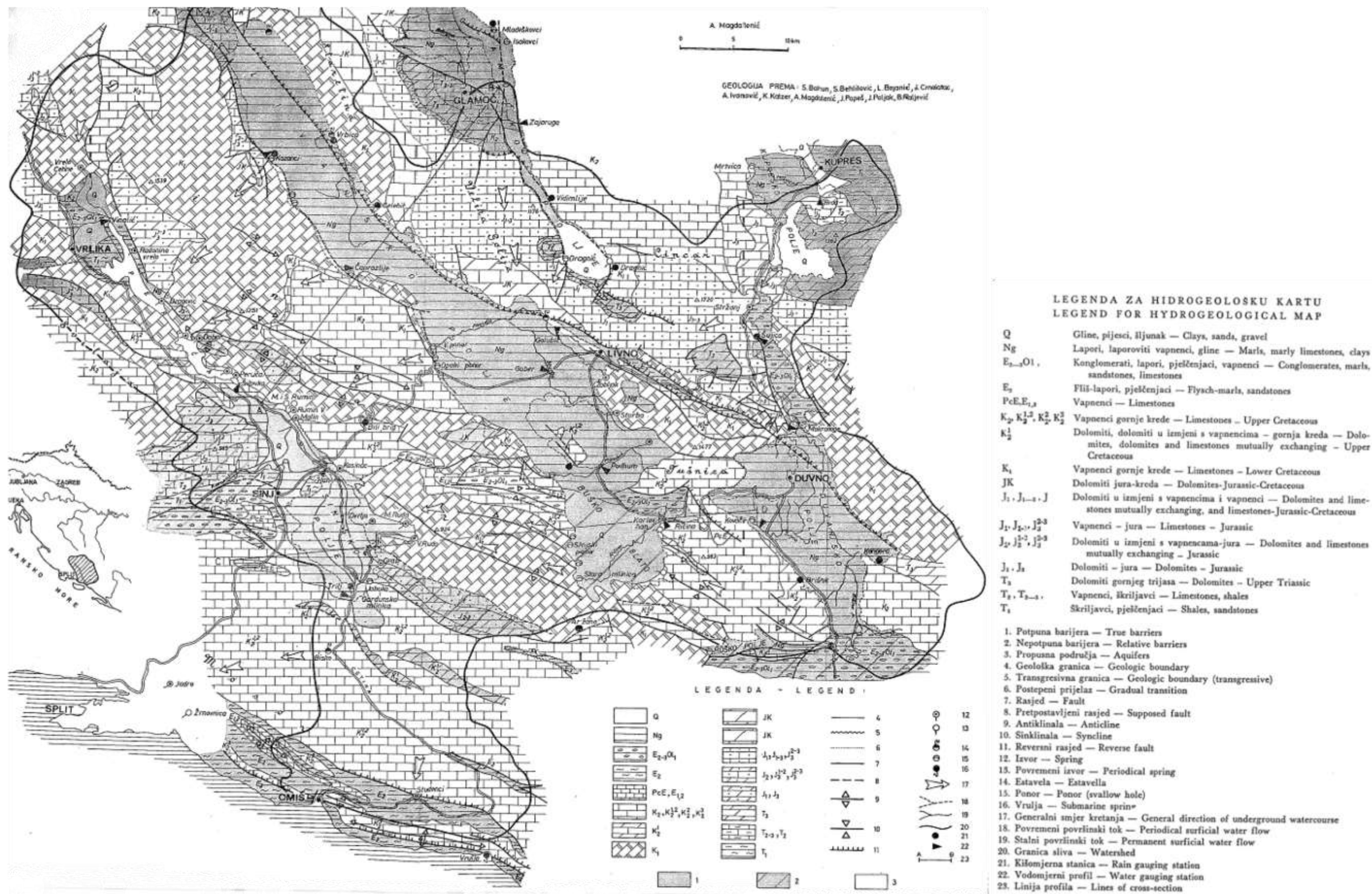
Slika 3.1. Hidrogeološka karta sliva (Banović, 2014.)
