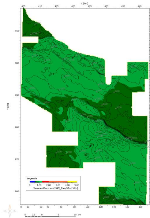
Slika 24.a) Zrelost prema Ro za “sloj” Kharita SR 1
