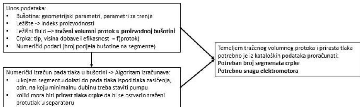
Slika 3-1. Prikaz algoritma u izračunu
