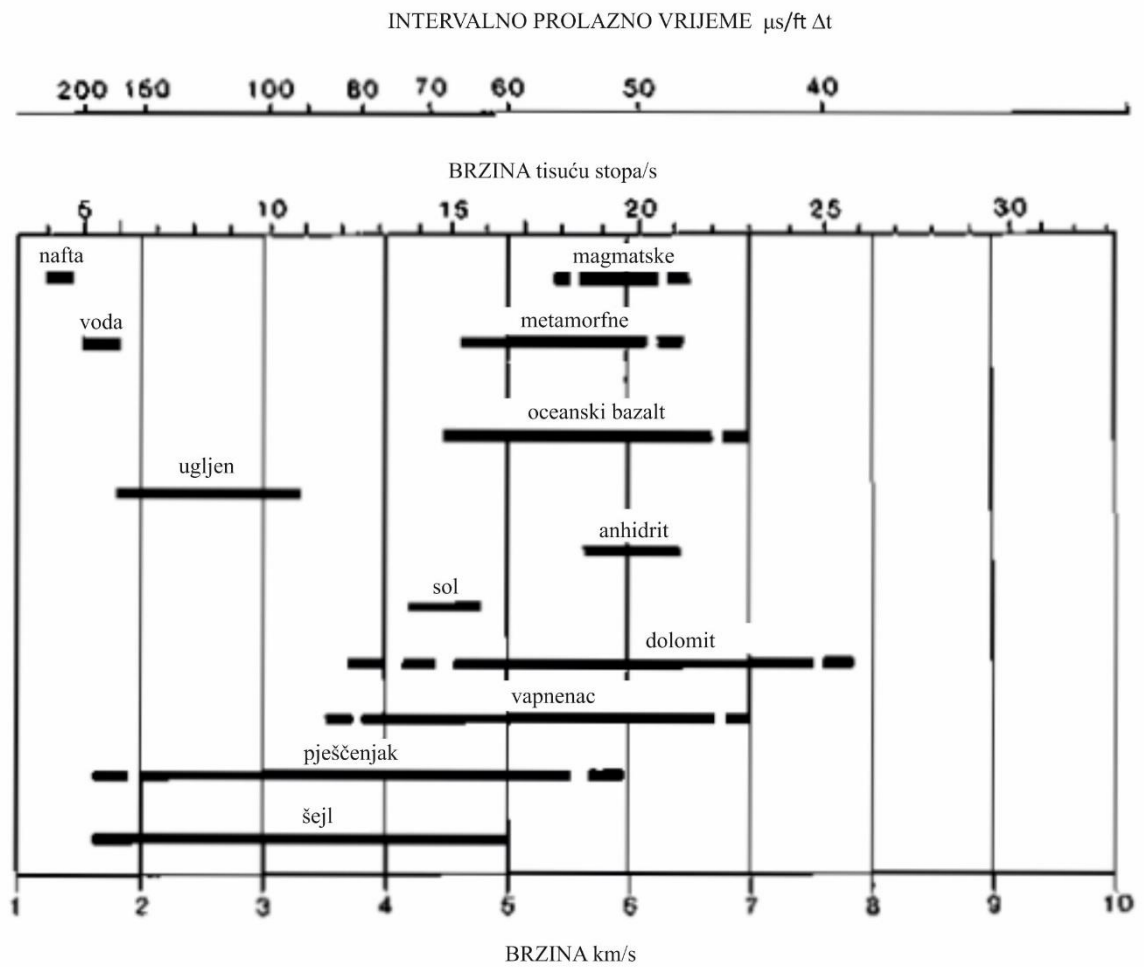
Slika 4-2. Prosječne brzine rasprostiranja valova u stijenama (ft – oznaka za stopu, a ona iznosi 0,3048 m) (Rider, 1996)
