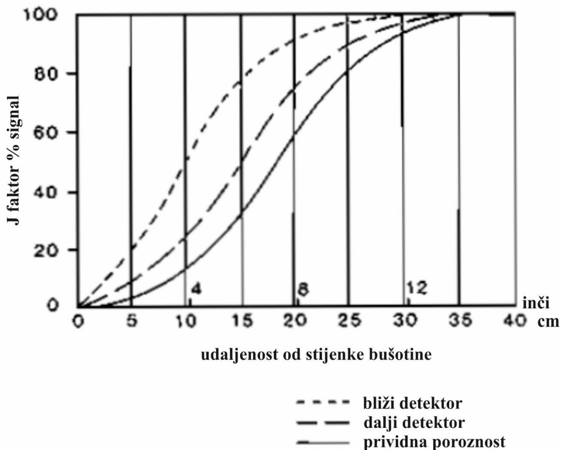
Slika 4- 6. Dubina prodiranja uređaja za neutronske karotaže (Rider 1996, modificirano prema Sherman i Locke, 1975)
