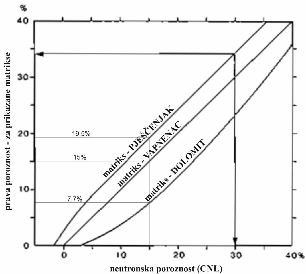
Slika 4- 5. Dijagram za korekciju ili procjenu poroznosti na temelju mjerenja neutronsom karotažom. (modificirano prema Schlumberger 1972; Rider 1996)
