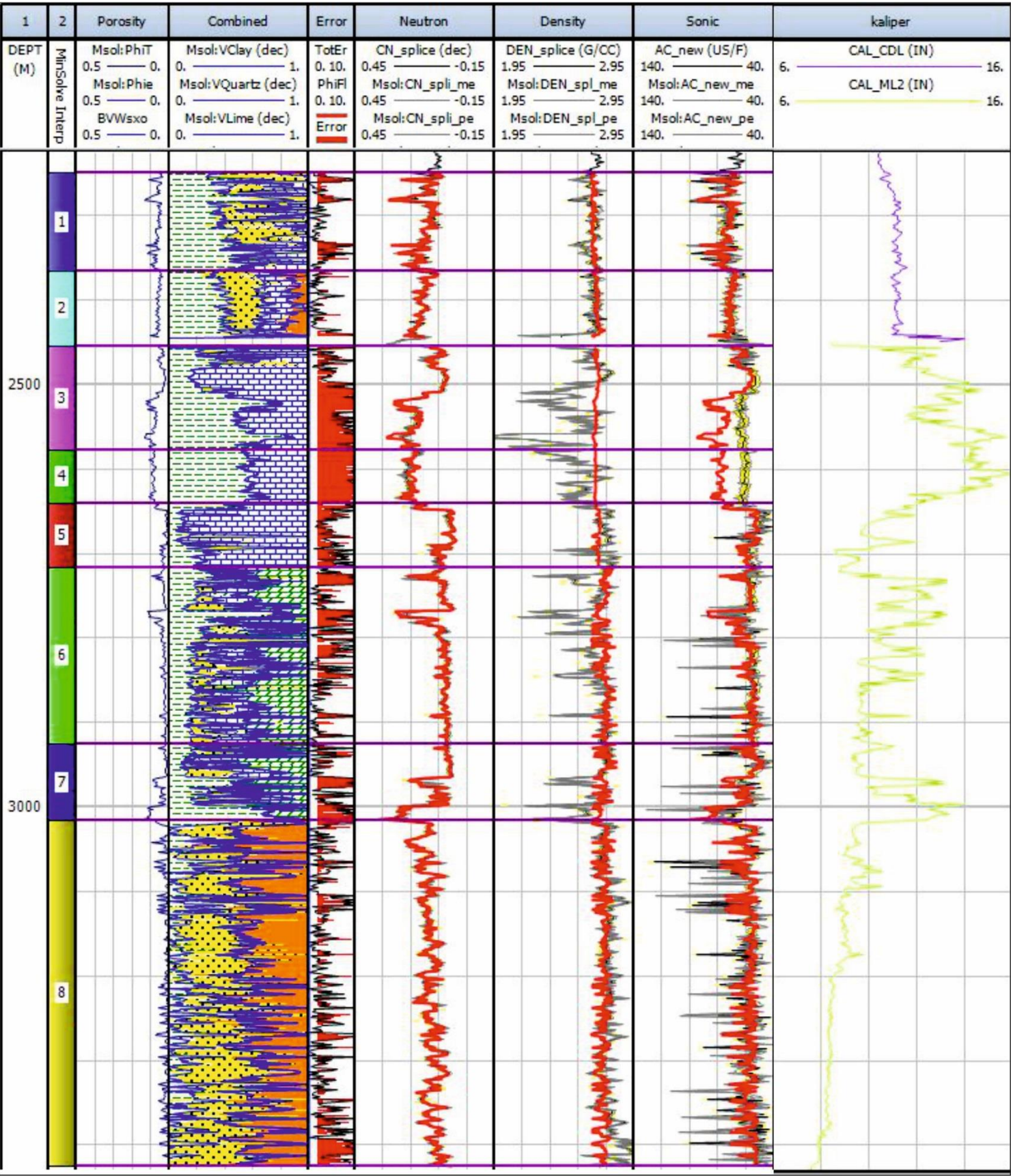
LEGENDA: kvarc glina kalcit muskovit dolomit
