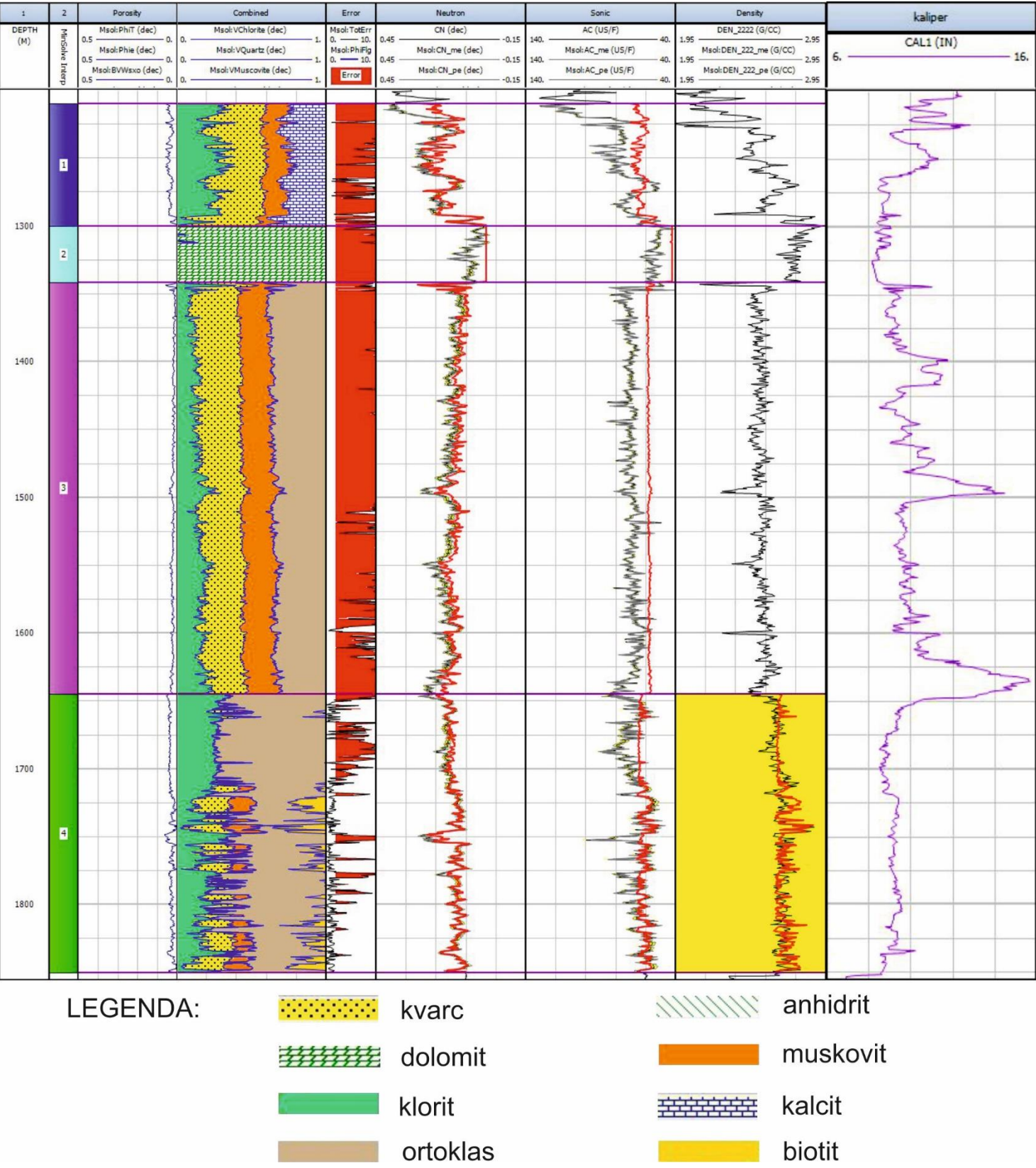
Slika 5-10. Procjena poroznosti za bušotinu 9. (1 – konglomeratični pješčenjak, 2 – anhidrit s tragovima karbonata, 3 – intruziv, 4 - škriljavac)
