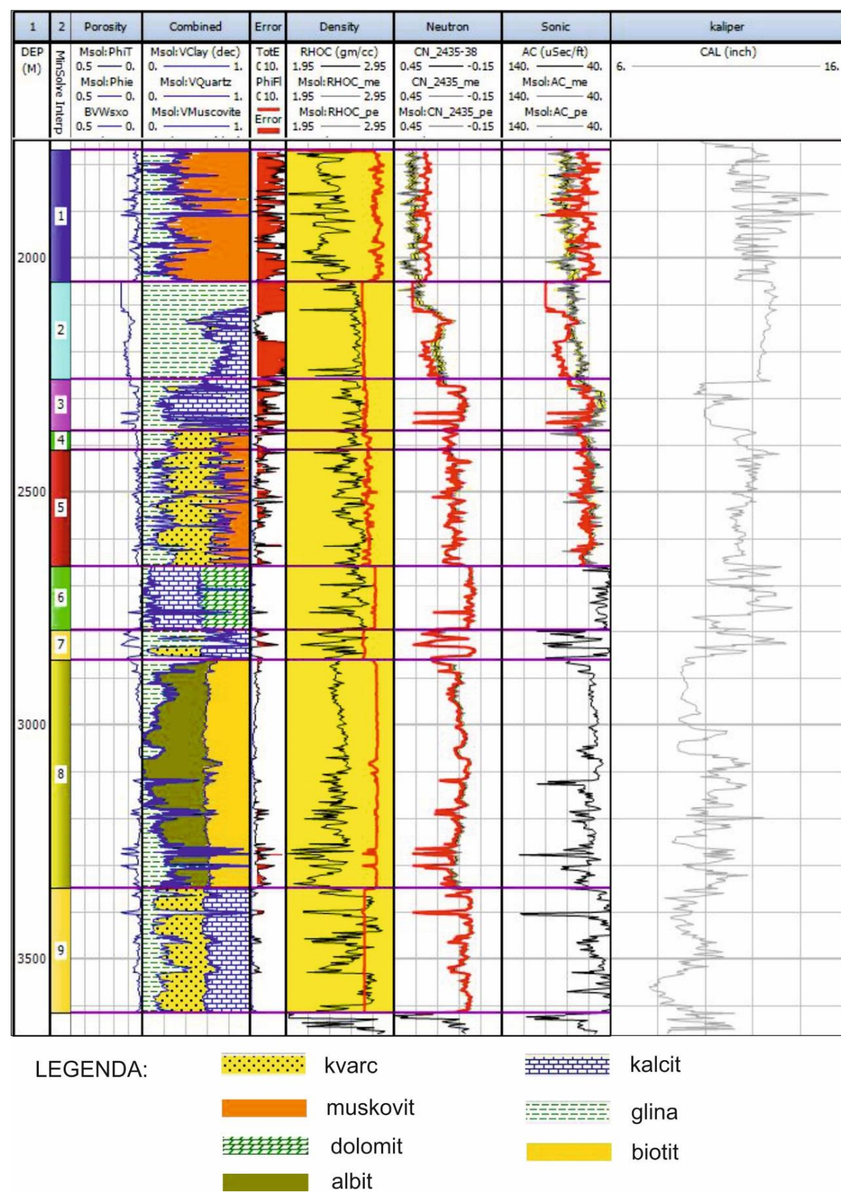
Slika 5-7. Procjena poroznosti za bušotinu 6. (1 – pješkovi lapor, 2 – lapor, 3 – brečokonglomerat, 4 – pješčenjak, 5 – konglomeratični pješčenjak, 6 – vapnenac, 7 – breča, 8 - tuf, 9 – breča)
