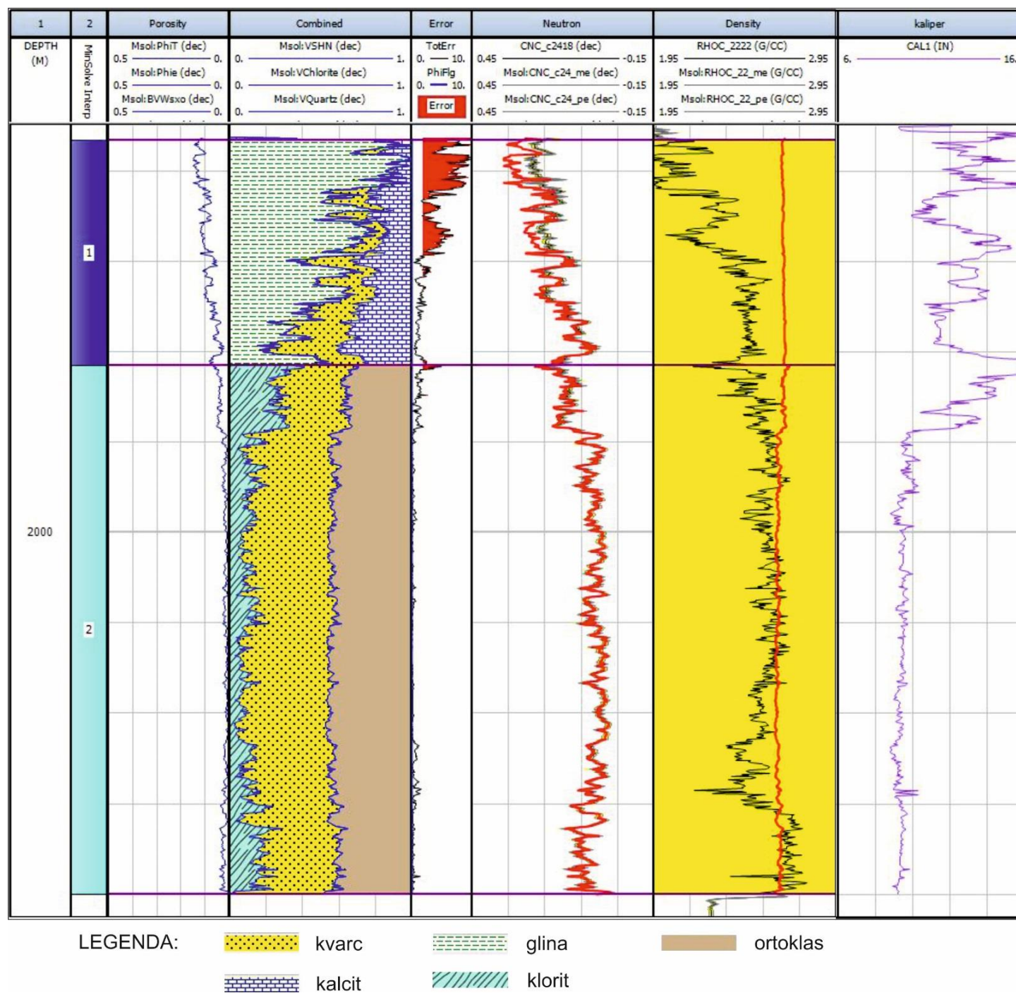
Slika 5- 4. Procjena poroznosti za bušotinu 3. (1 – breča, 2 – škriljavac)
