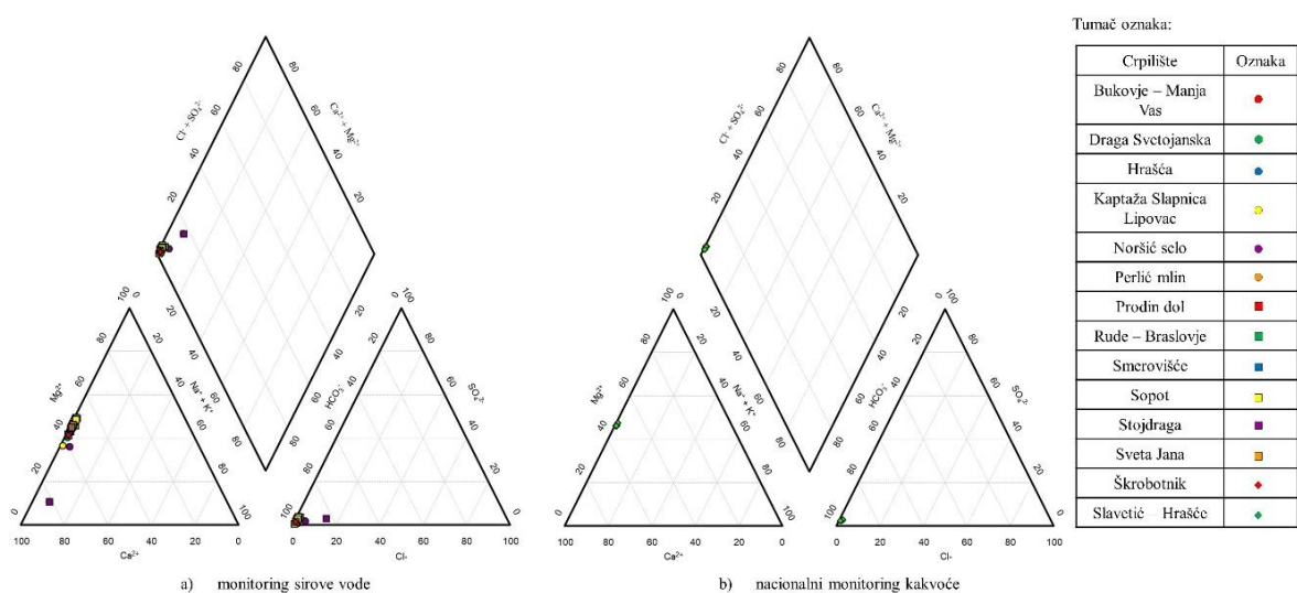
Slika 7-16. Piperovi dijagrami GTPV-a Žumberak – Samoborsko gorje
