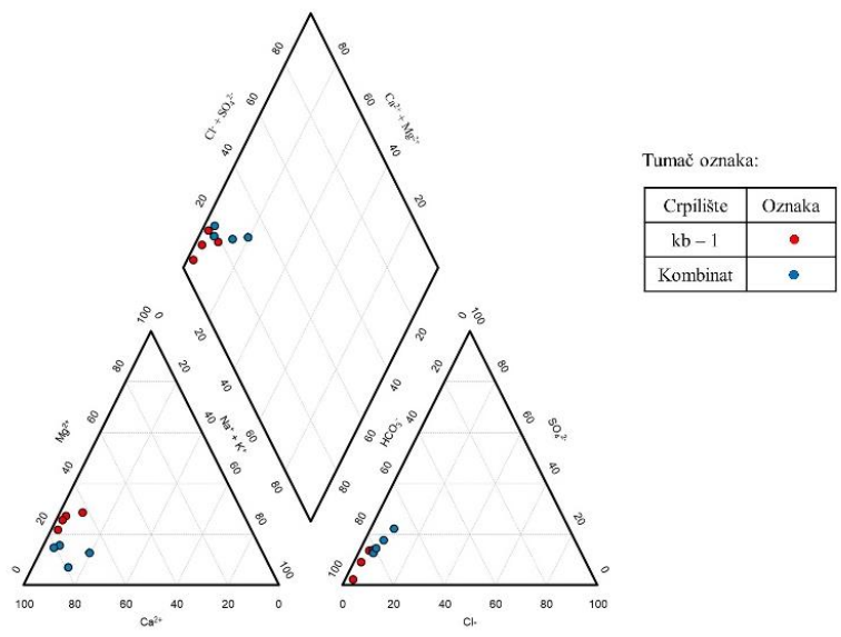
Slika 7-18. Piperov dijagram GTPV-a Donji tok Une
