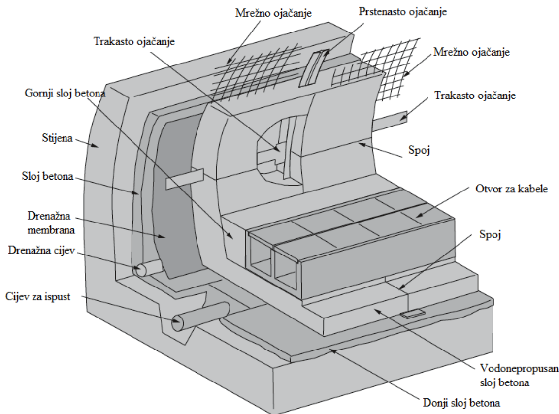
Slika 2-30 Drenaža podzemne željeznice (Kolymbas, 2008.)
