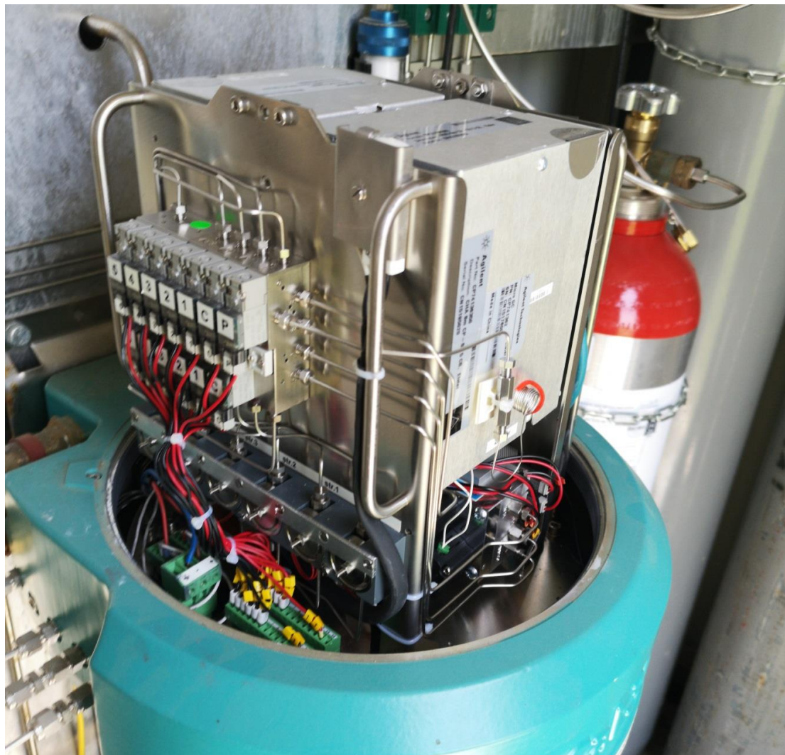
Slika 5-5. Kromatograf EnCal 3000
