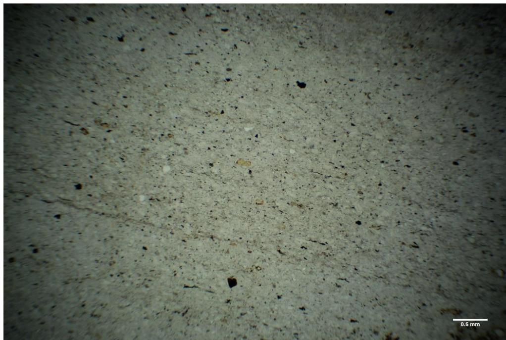
Slika 4-8. Mikropetrografski izbrusak, UZORAK Slap-3 (paralelni nikoli) → vitriklastični tuf građen od dobro sortiranih krhotina vulkanskoga stakla
