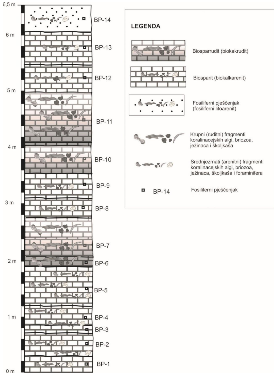
Slika 4-1. Prikaz sedimentnog slijeda Bela Pećina (uzorci s oznakom BP-1 do BP-14)
