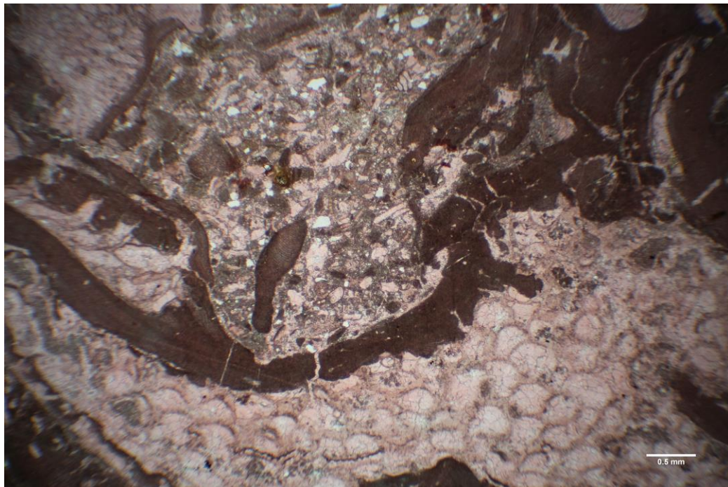
Slika 4-7. Mikropetrografski izbrusak, UZORAK T-5-7 (pararelni nikoli) → biosparrudit građen od dobro zaobljenih bioklasta koralinacejskih algi te iznimno krupnih fragmenata briozoa; moguća inkrustacija koralinacejskim algama i briozoima. U prostoru između skeleta nalazi se matriks sastavljen od mikrita, sitnozdrobljenog kršja i silicilasta.
