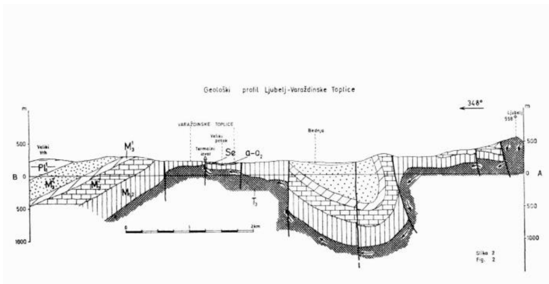
Slika 2-1. Geološki profil kroz naslage okolice Varaždinskih Toplica (ŠIMUNIĆ, 1988)
