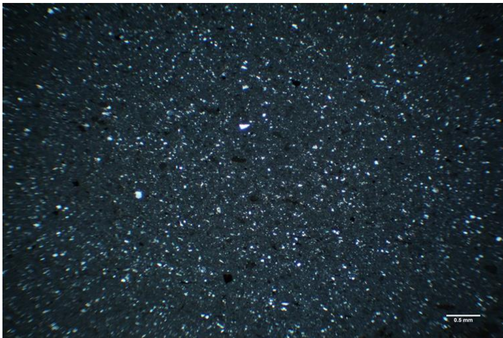
Slika 4-9. Mikropetrografski izbrusak, UZORAK Slap-3 (ukriženi nikoli)
