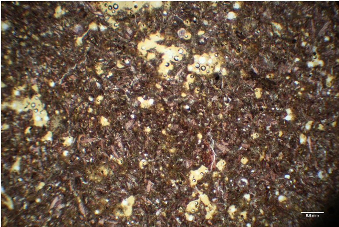
Slika 4-10. Mikropetrografski izbrusak, UZORAK AM-1 (paralelni nikoli) → biomikrit sastavljen dominantno od sitnih planktonskih foraminifera u mikritnoj osnovi.
