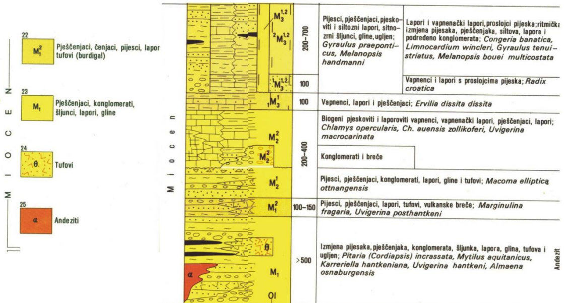
Slika 2-2. Isječak OGK 1 : 100 000, list Varaždin (ŠIMUNIĆ i dr., 1983)
