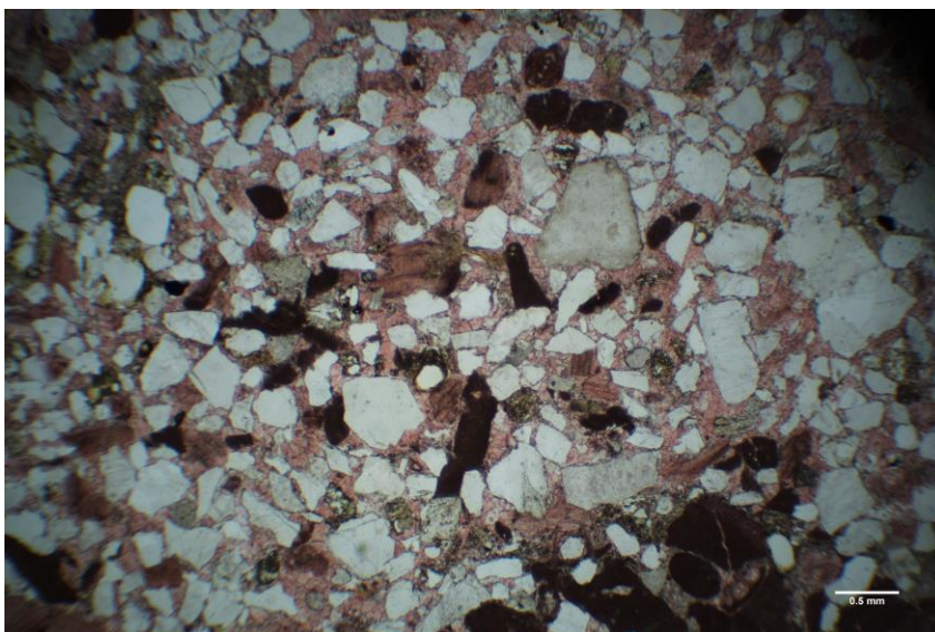
Slika 4-5. Mikropetrografski izbrusak, UZORAK BP-14 (paralelni nikoli) → fosiliferni pješčenjak građen dominantno od siliciklastičnog detritusa s česticama kvarca, litoklastima metamornih stijena te feldspata; podređeno su prisutni bioklasti koralinacejskih algi te bentičke foraminifere
