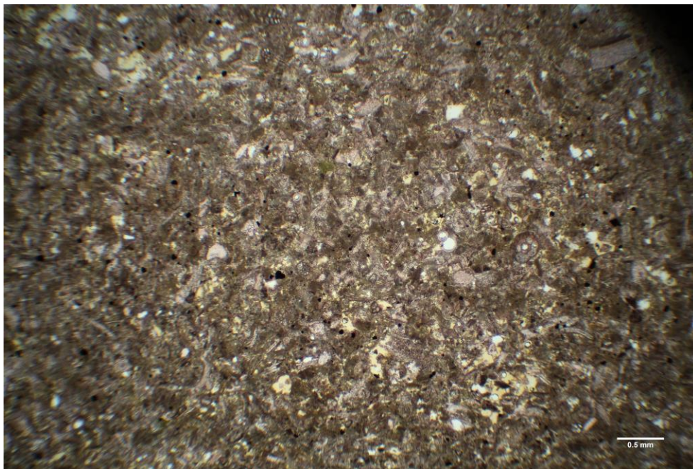
Slika 4-12. Mikropetrografski izbrusak, UZORAK AM-3 (paralelni nikoli) → biomikrit građen od fosila planktonskih foraminifera i mikrita; podređena pojava fragmenata ježinaca.
