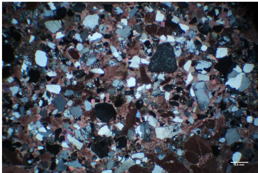
Slika 4-6. Mikropetrografski izbrusak, UZORAK BP-14 (ukriženi nikoli) → fosiliferani pješčenjak
