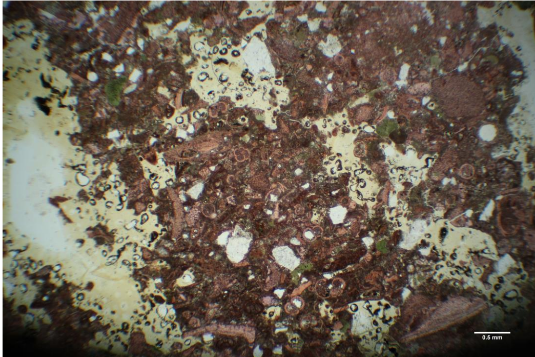
Slika 4-13. Mikropetrografski izbrusak, UZORAK AM-4 (paralelni nikoli) → biomikrit građen dominantno od ljušturica fosila planktonskih foraminifera; niži udio fragmenata ježinaca različitih veličina, te nizak udio siliciklastičnog materijala poput kvarca; čestice glaukonita (zelene boje) također su zastupljene u uzorku.
