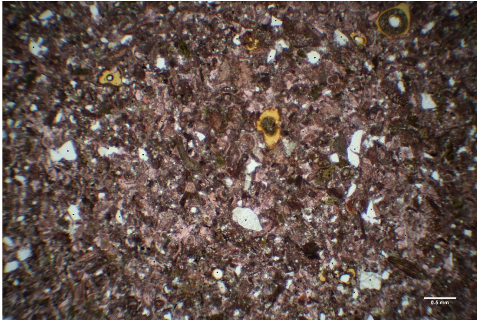
Slika 4-11. Mikropetrografski izbrusak, UZORAK AM-2 (paralelni nikoli) → biomikrit primarno građen od sitnih ljušturica planktonskih foraminifera u mikritnoj osnovi te nerijetka pojava glaukonita (zelene boje)
