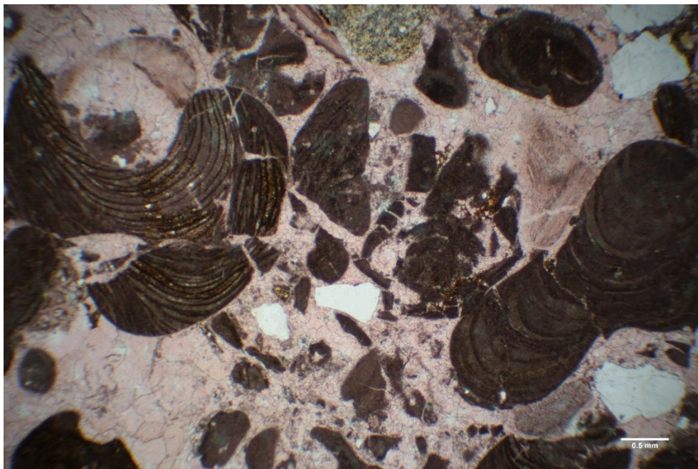
Slika 4-3. Mikropetrografski izbrusak, UZORAK BP-13 (paralelni nikoli) → biosparrudit s bioklastima koralinacejskih algi te podređeno fragmentima ježinaca i česticama kvarca
