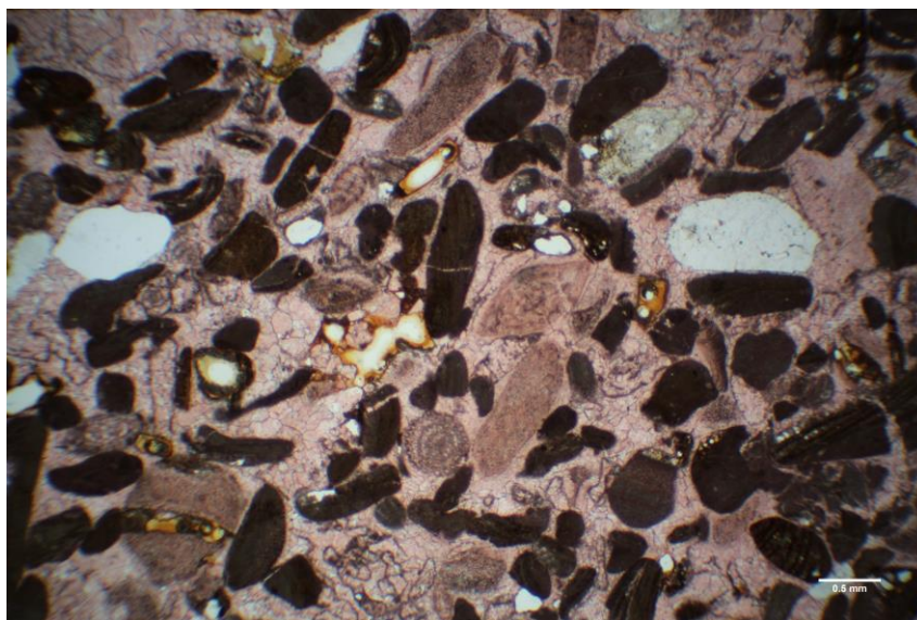
Slika 4-4. Mikropetrografski izbrusak, UZORAK BP-3 (paralelni nikoli) → biosparit građen od dobro sortiranih bioklasta koralinacejskih algi (< 2 mm) i detritusa ježinaca, školjkaša i foraminifera
