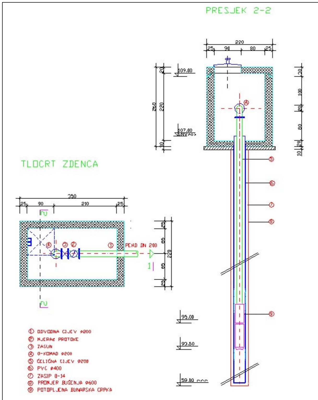
Slika 3.44: Shematski prikaz izvedbe zdenca Interventnog crpnog sustava
