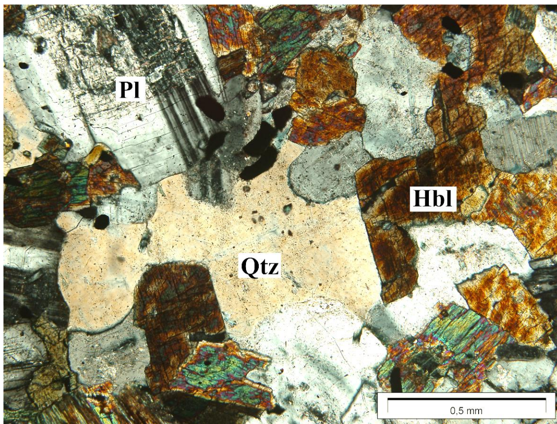
Slika 7.44 Plagioklas (Pl), hornblenda (Hbl) i intersticijski kvarc (Qtz) u hornblenda monzodioritu. Obod-34, J-21, interval 2475 – 2476,3 m. N+
