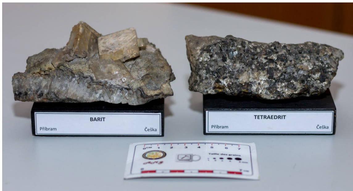
Slika 4-14. Barit i tetraedrit
