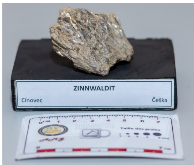
Slika 4-3. Zinnwaldit
