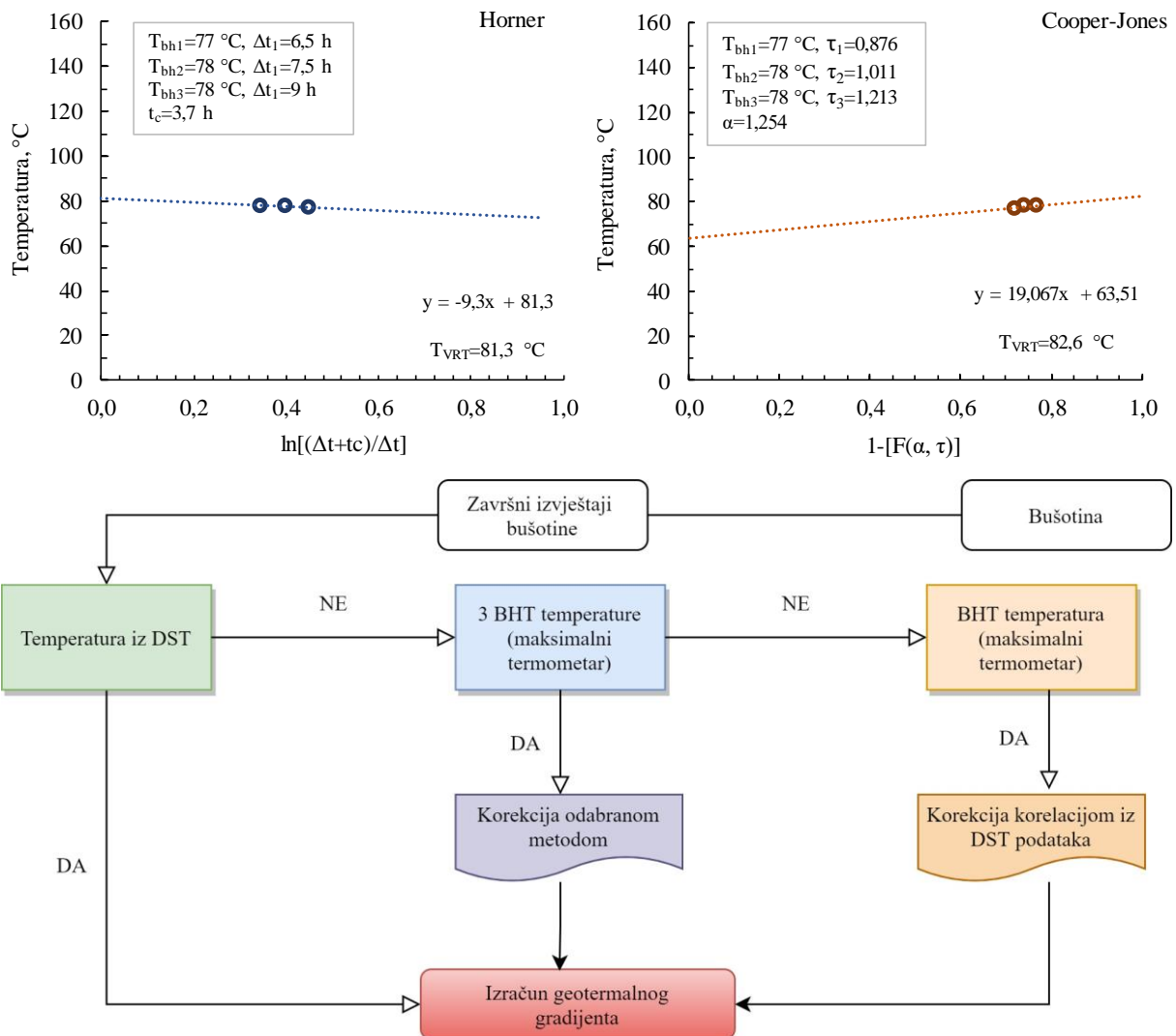
Slika 5.2. Primjer određivanja statičke temperature metodom Horner i Cooper-Jones za bušotinu Hrvatsko zagorje-1 na dubini 2595 m (za usporedbu T_{DST} @ 2370 \text{ m}=102 \text{ °C} ) i postupak određivanja geotermalnog gradijenta
