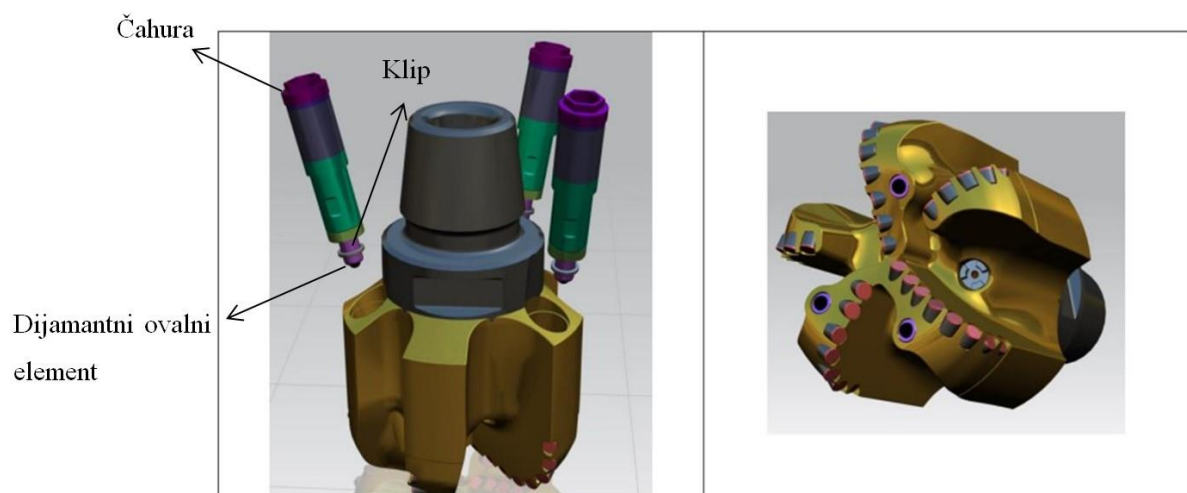
Slika 3-1. Smještaj kontrolnih mehanizama za podešavanje dubina prodiranja reznih elemenata u stijenu (Jain et al., 2016)
