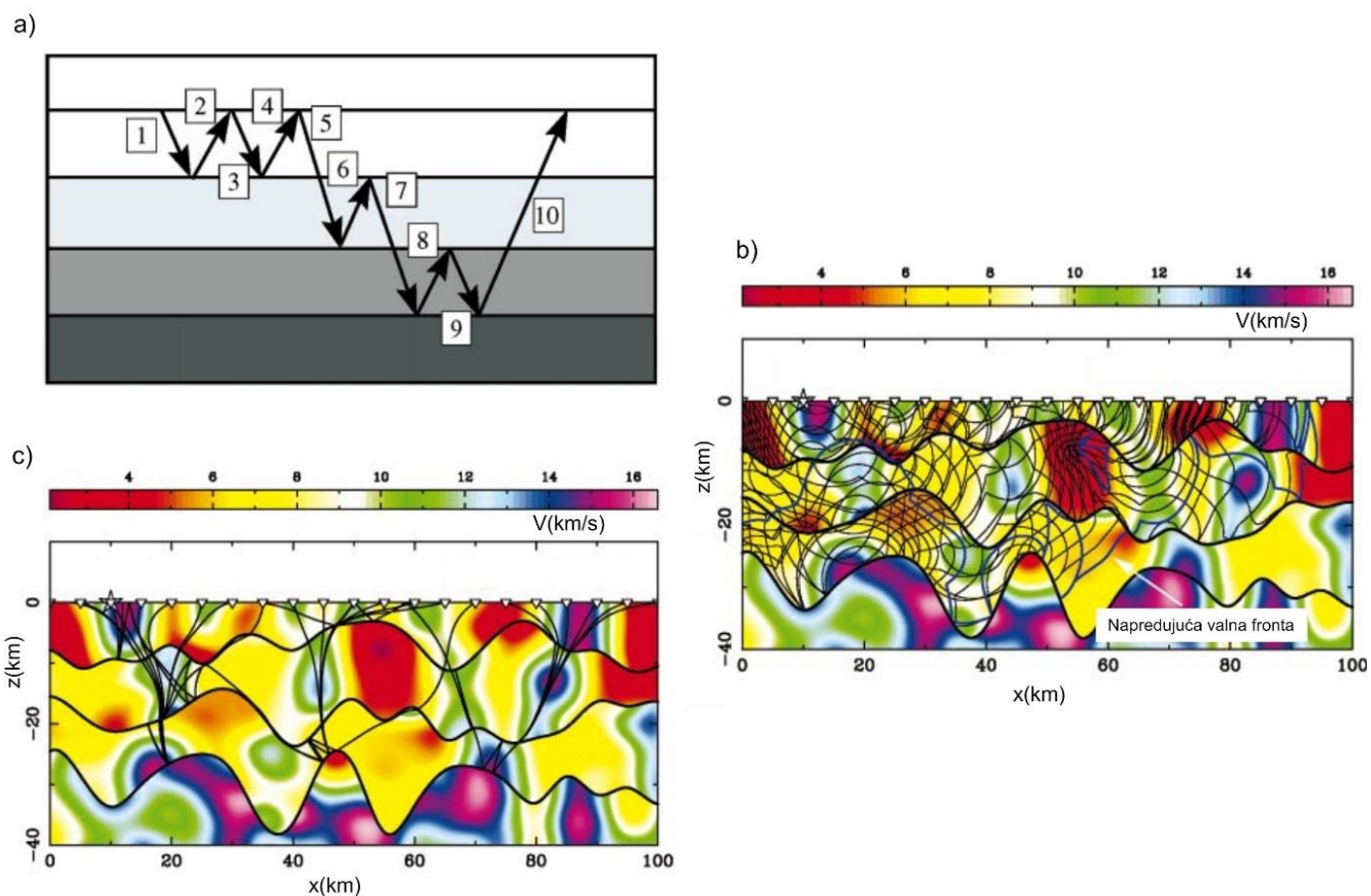
Slika 4.16 Trasiranje nailaska višestrukog refleksa u modelu s velikim lateralnim promjenama brzine i dubine slojeva. a) deset grana višestrukog refleksa b) napredovanje vala prikazano je valnim frontama u intervalima 0,4 sekunde (takne linije) c) valne zrake višestrukog refleksa od izvora na površini (zvjezdica) do prijemnika – trokutići (Rawlinson i Sambridge 2004b).
