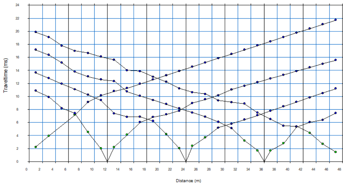
Slika 5.8. Graf „vrijeme – brzina“ dobiven pikiranjem prvih nailazaka (SRS-Hruškovec)
