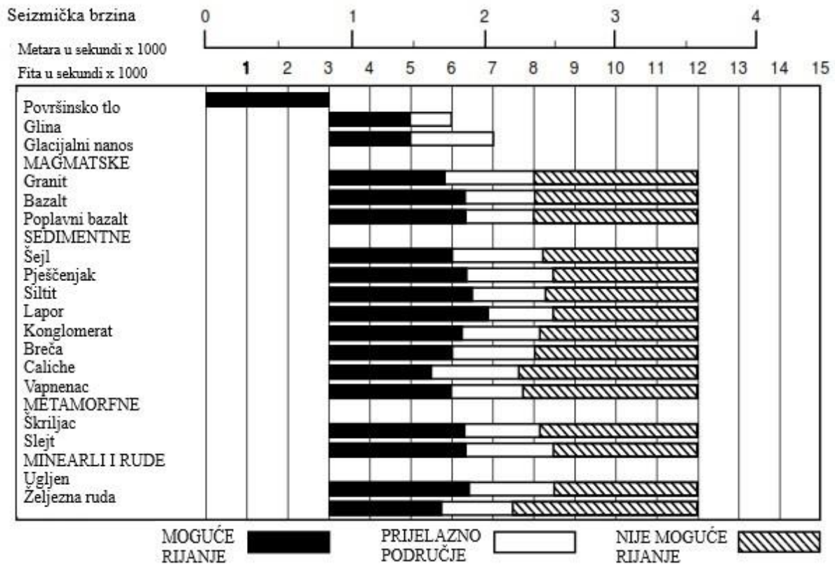
Slika 4.20. Dijagram za procjenu mogućnosti otkopavanja stijenske mase metodom rijanja dozerom Caterpillar D8R (Caterpillar, 2015)
