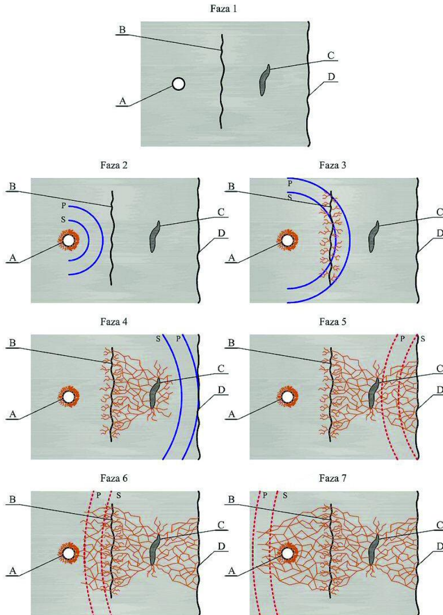
Slika 4.7. Shematski prikaz teorije jezgre ili valova naprezanja i pukotina: A – mitska bušotina, B – vlakna pukotina, C – oštećenje, D – slobodna površina, P – longitudinalni val, S – transverzalni val (Ester, 1996; Antičević, 2011)
