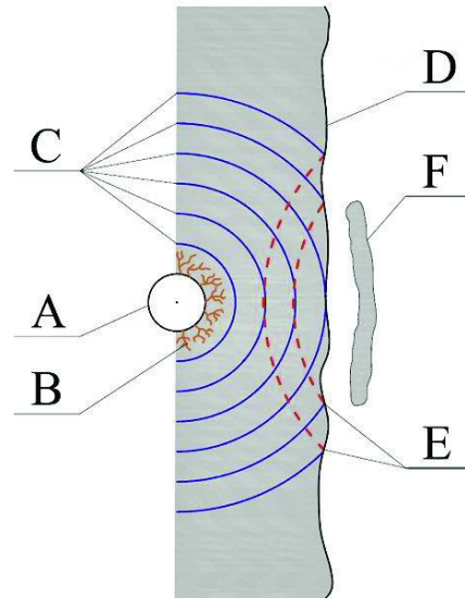
Slika 4.5. Osnovni koncept teorije refleksije: A – minsku bušotina, B – zona drobljenja, C – širenje tlačnog vala, D – slobodna površina, E – reflektirani (vlačni) val, F – odlomak dijela stijene na slobodnoj površini (Ester, 1996; Antičević, 2011)
