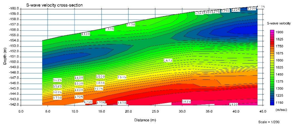
Slika 5.10. MASW – terensko snimanje i obrada snimljenih podataka (Jug i sur., 2020)
