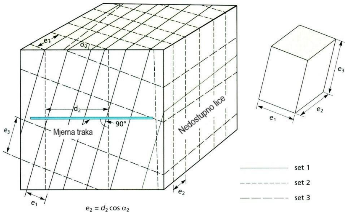
Slika 2.3. Mjerenje razmaka diskontinuiteta opažanjem izdanaka stijena na površini (ISRM, 1981)
