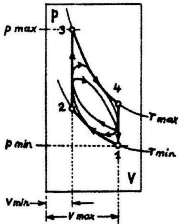
Slika 3-3. Realni indikatorski dijagram (Košćak Kolin, 2000)
