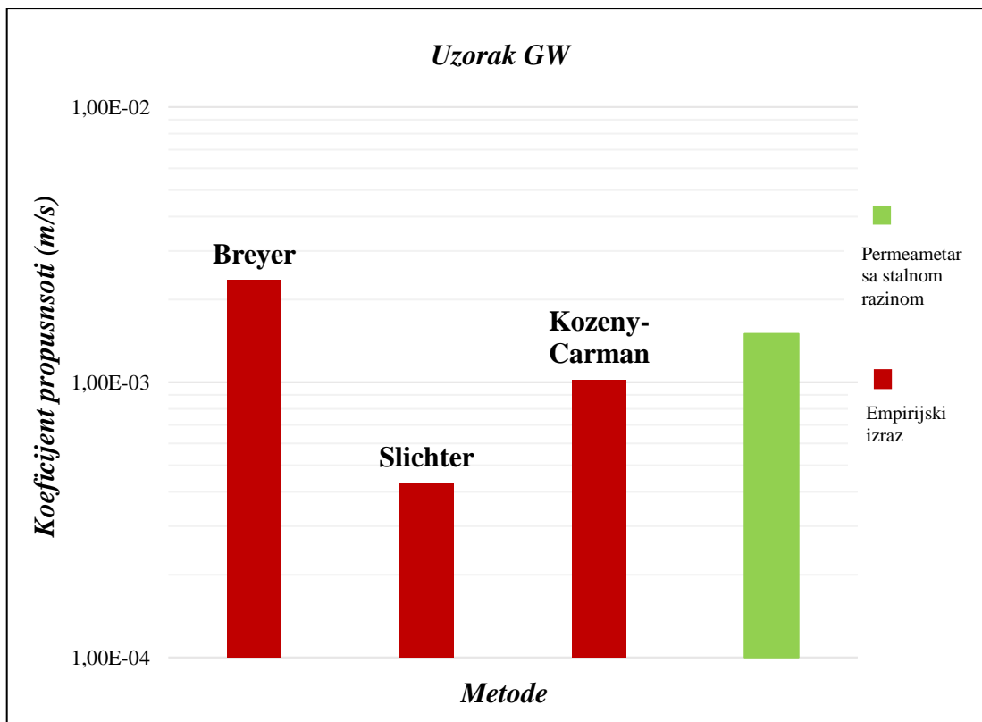
Slika 7-3. Usporedba vrijednosti koeficijenta propusnosti za uzorak GW
