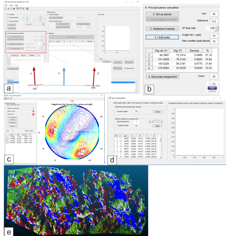
Slika 4-5 Polu-automatsko identifikacija setova diskontinuiteta u softveru DSE : a) test koplanarnosti; b) statistička analiza; c) stereografska projekcija polova normala diskontinuiteta; d) uređivanje clusters ; e) prikaz identificiranih setova diskontinuiteta (Riquelme et al., 2014.).
