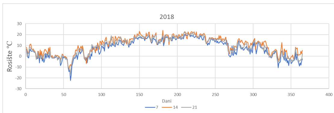
Slika 3-1 kretanje rosišta 2018
