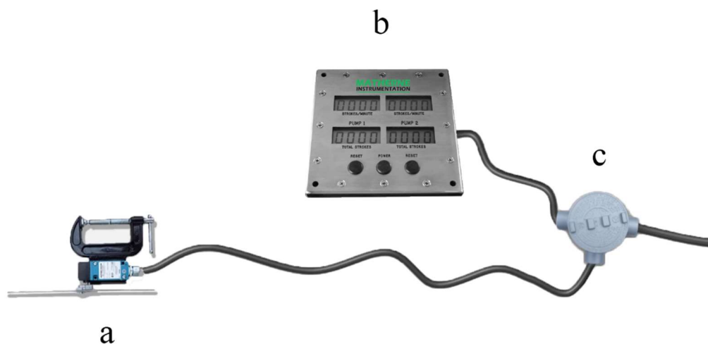
Slika 2-9. Shema sustava mjerenja broja hodova isplačne sisaljke (Matherne Instrumentation, 2017 b)
