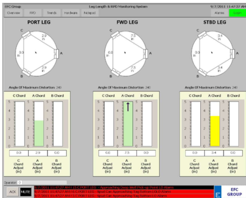
Slika 4-3. Softver za praćenje stanja nogu samopodižuće platforme (Electro-Flow-Controls, 2020)
