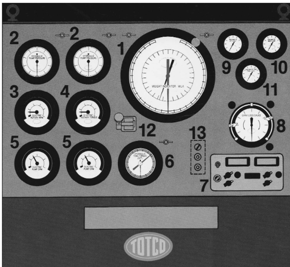
Slika 3-3. Shema instaliranih indikatora na tipičnoj konzoli (Totco, 1980)
