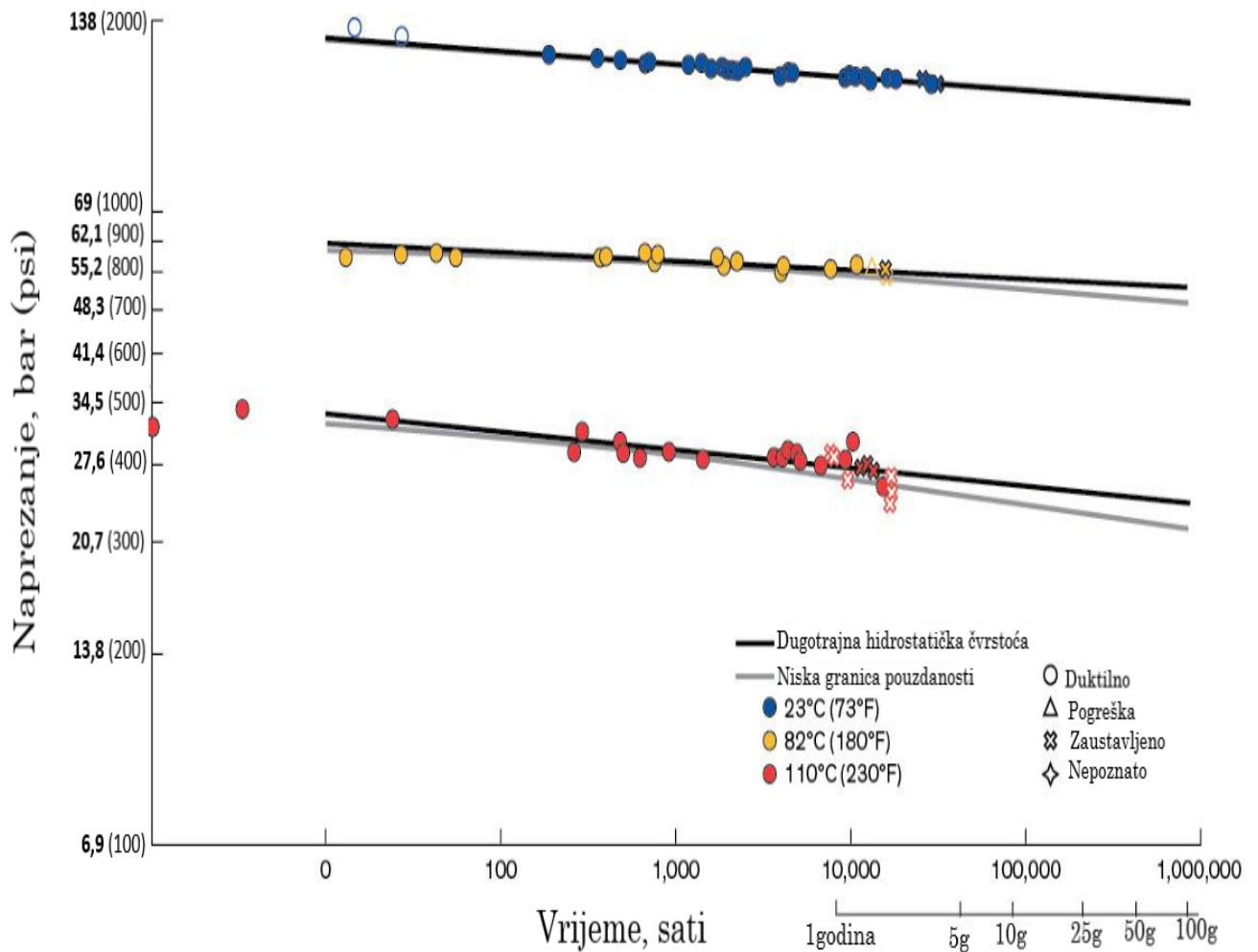
Slika 2-4. Ovisnost naprezanja bimodalnog HDPE materijala o vremenu za različite radne temperature (Chang i Baker, 2016)
