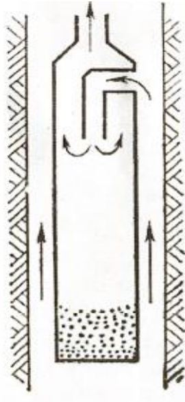
Slika 4 - 4. Neizravno pješčano sidro (Zelić i Čikeš, 2006)
