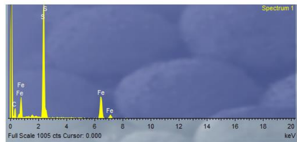
Slika 60. Energetsko disperzivni spektar zrna pirita iz uzorka tinjčevog škrljavca oznake 402/12.
