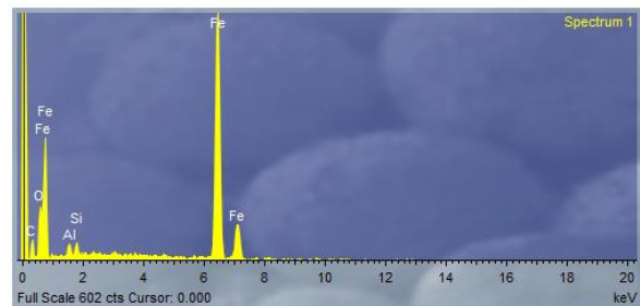
Slika 61. Energetsko disperzivni spektri zrna hematita iz uzorka tinjčevog škrljavca oznake 402/12.
