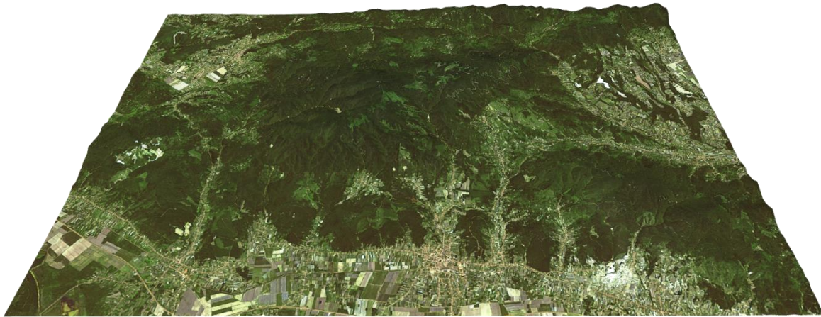
Slika 2. 3D prikaz reljefa Psunja. Nadmorska visina je dvostruko uvećana (RGB snimak je izveden iz Landsat 8 pojaseva ( Landsat Science, 2015 ), dok je 3D prikaz dobiven Qgis2threejs ( Akagi, 2020 ) dodatkom za QGIS ( QGIS Development Team, 2019 )).
