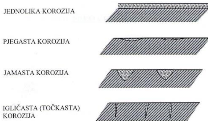
Slika 3-10. Različiti tipovi korozije (Stupnišek-Lisac, 2007).
