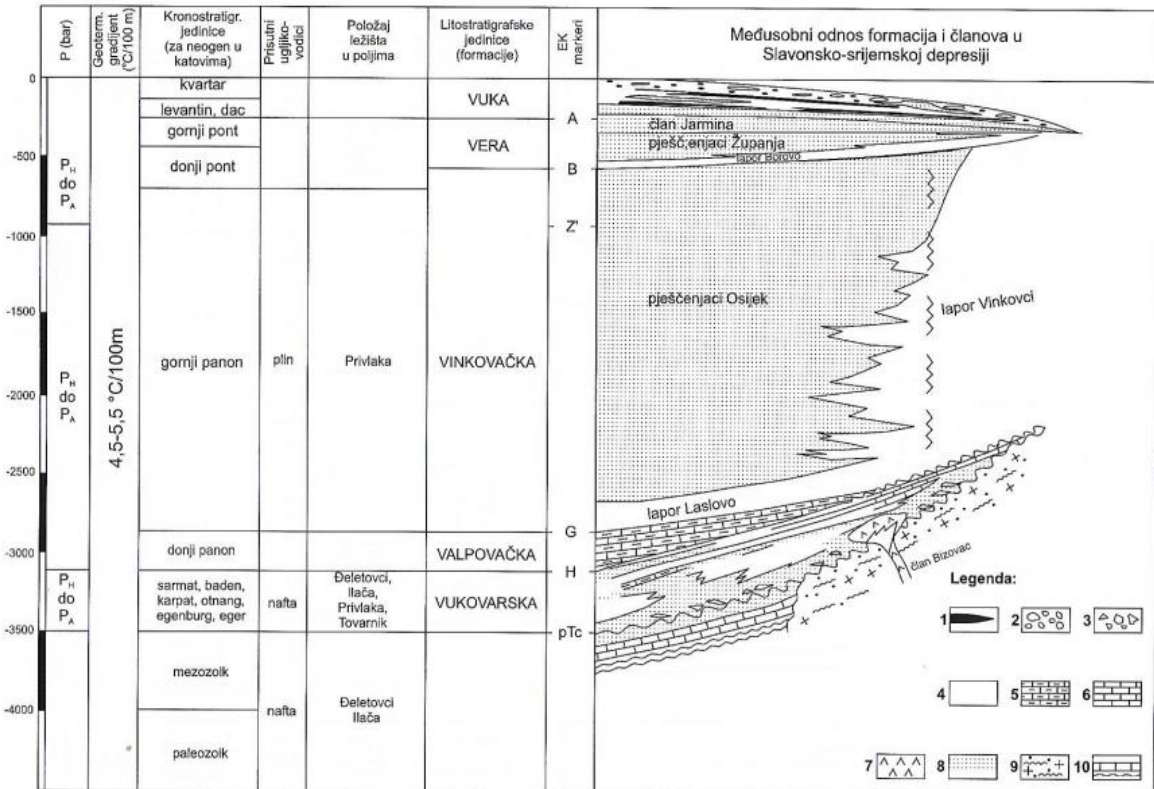
Slika 2-2. Stratigrfske jedinice, litoški sastav i položaj važnijih ležišta u Slavonko-srijemskoj depresiji; često se koristi i za najistočniji dio Dravske depresije (modificirano prema Velić, 2007)
