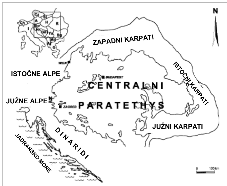
Slika 3-1. Smještaj centralnog Paratethysa (prilagođeno prema Pavelić 2002)
