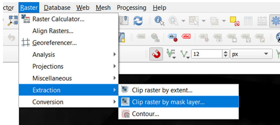
Slika 3-13 Clip raster
