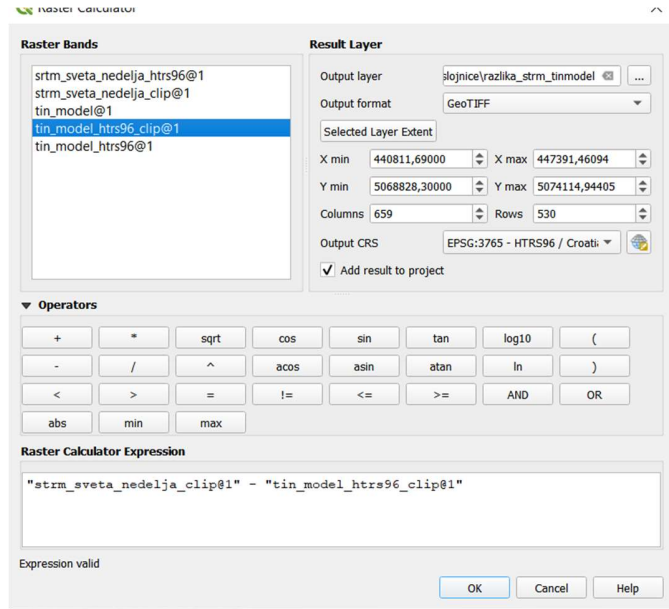
Slika 3-15 Raster Calculator
