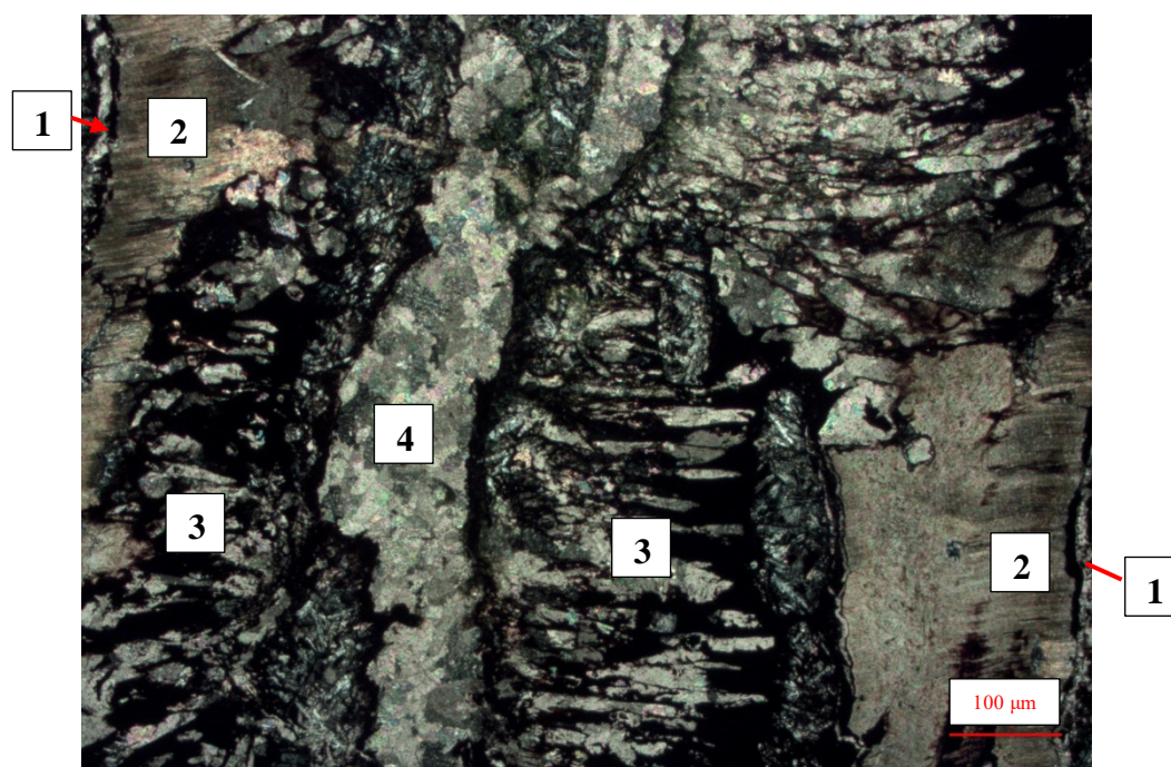
Slika 5-16. Mikrofotografija uzoraka MVIM 21B2 (N+). Prikaz žile koncentrične građe.
