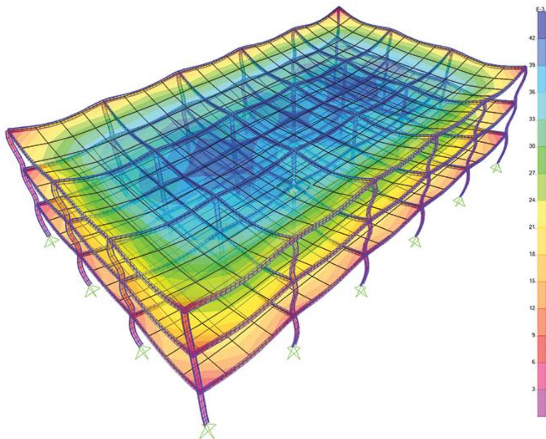
Slika 2-8 Prikaz rezultata naprežanja konstrukcije u SAP2000 programu (Csi America, 2020)
