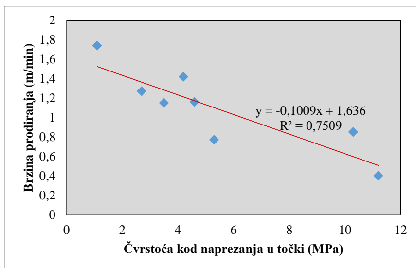
Slika 4-4. Ovisnost brzine prodiranja bušaćeg alata kroz stijenu o indeksu čvrstoće stijene kod naprezanja u točki
