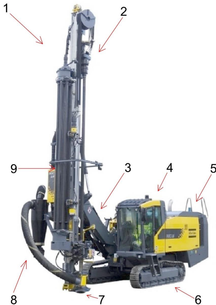
Slika 3-1. Osnovni dijelovi bušilice (Atlas Copco, 2010.)
