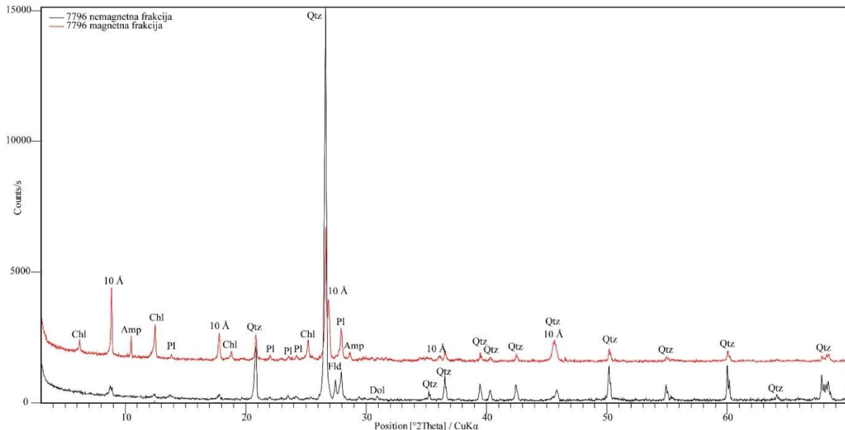
Slika 6-9. Difrakcijska slika magnetski separiranog uzorka H-3 (crno - nemagnetna frakcija; crveno - magnetna frakcija).
