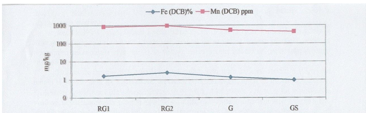
Slika 15 - Koncentracija topivog željeza i mangana u uzorcima poplavnih sedimenata Rudarske Gradne i Gradne, DCB - ditionit-citrat-bikarbonat, (Čović, 2003)
