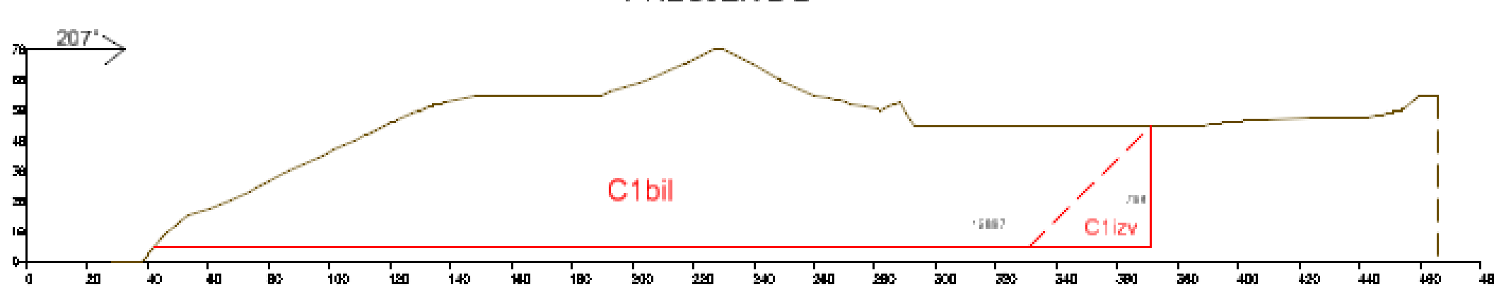
PRESJEK 2-2'
