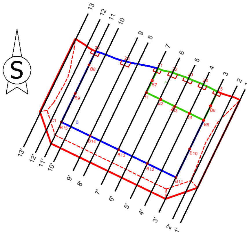
Slika 5-2-2-a. Presjeci u karakterističnim točkama
