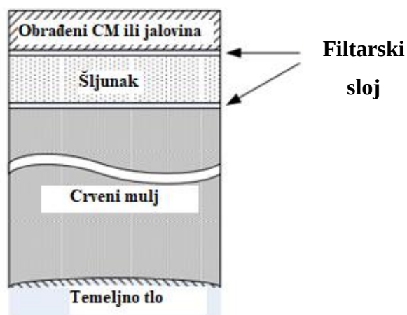
Slika 3-1. Skica slojeva završnog pokrova na lokaciji saniranog kopa (Aluminium of Greece, 2006)
