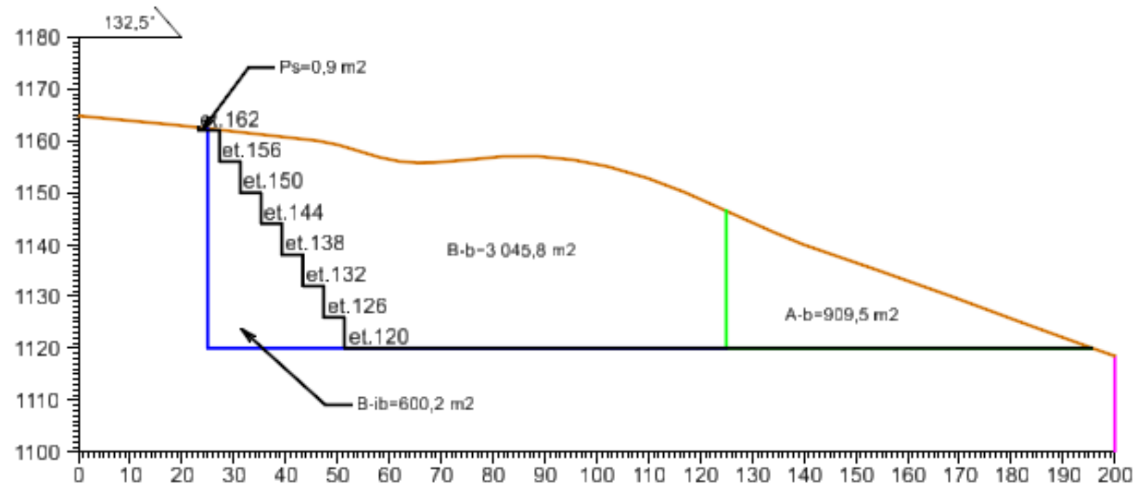
Presjek 5-5'
