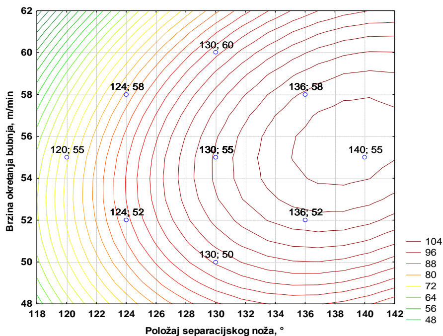
Slika 4 – 213 Nivo-linije regresijske plohe ovisnosti kvalitete koncentrata klase 2/1 mm o brzini okretanja bubnja i položaju separacijskog noža – grupa „TP“
