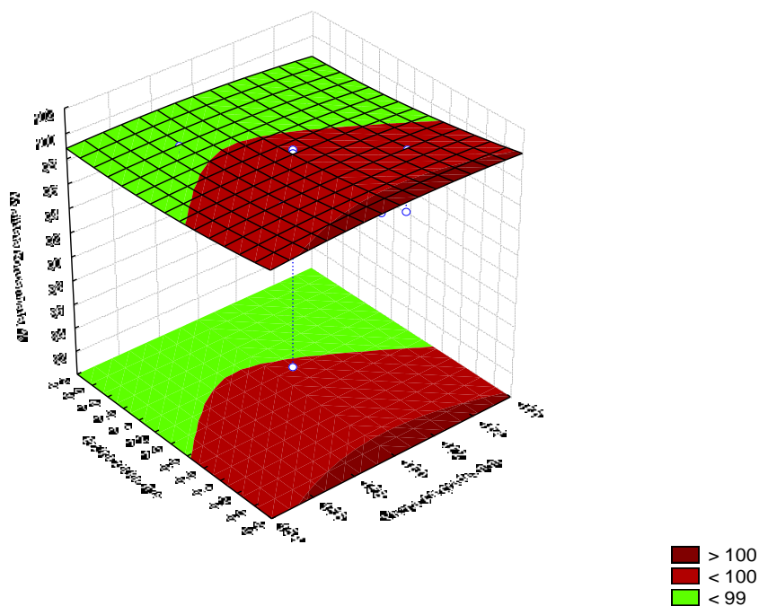
Slika 4 – 200 Regresijska ploha ovisnosti kvalitete koncentrata klase 1/0,5 mm o brzini zraka i visini pregrade – grupa „TP“
