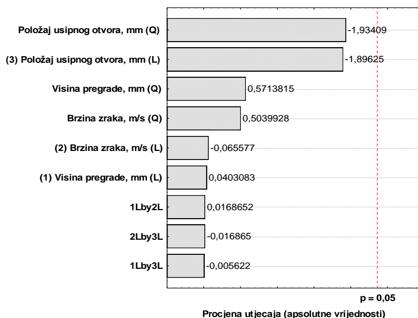
Grafikon 4 – 13 Procjena veličine utjecaja radnih parametara i njihovih međudjelovanja na kvalitetu koncentrata klase 1/0,5 mm – grupa „OSKKŽ“
