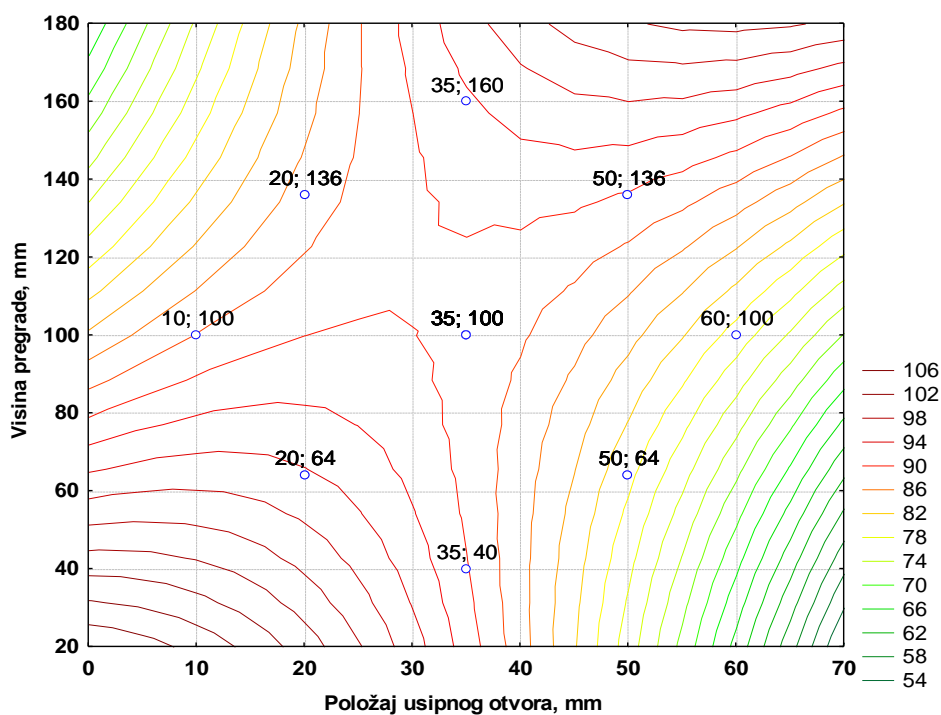
Slika 4 – 45 Nivo-linije regresijske plohe ovisnosti kvalitete koncentrata klase 2/1 mm o visini pregrade i položaju usipnog otvora – grupa „Z“
