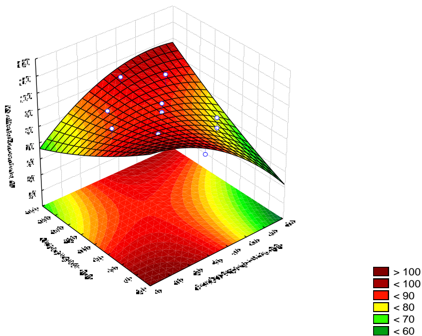
Slika 4 – 44 Regresijska ploha ovisnosti kvalitete koncentrata klase 2/1 mm o visini pregrade i položaju usipnog otvora – grupa „Z“
