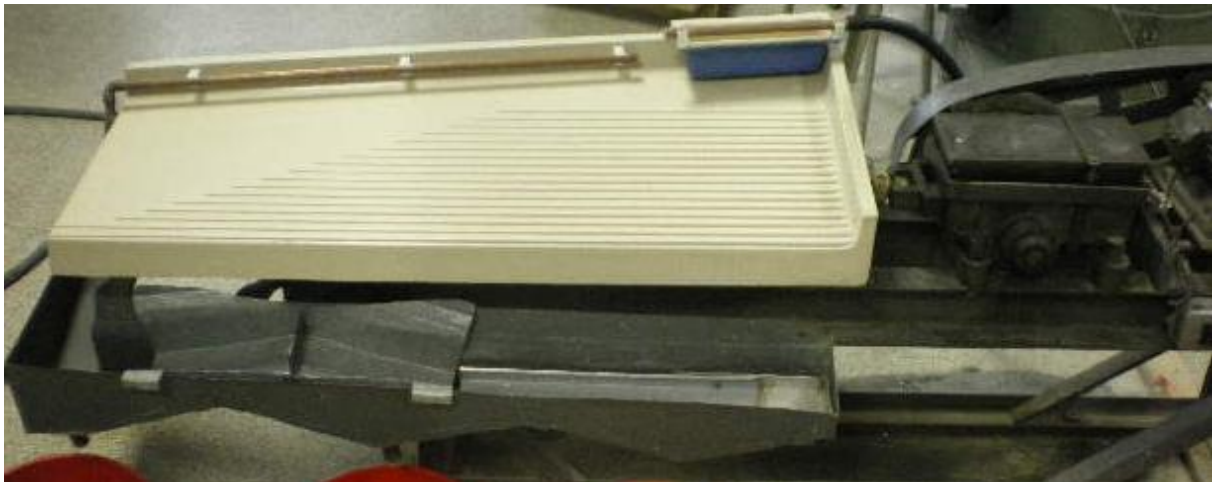
Slika 4 – 25 Koncentracijski stol Wilfley
