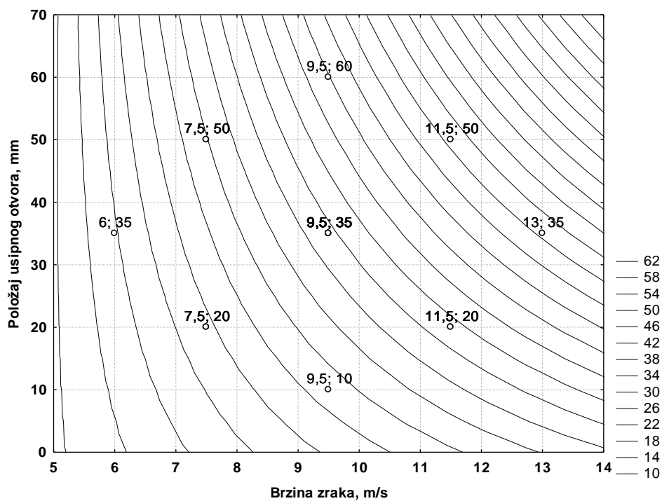
Slika 4 – 77 Nivo-linije regresijske plohe ovisnosti masenog iskorištenja klase -0,5 mm o položaju usipnog otvora i brzini zraka – grupa „Z“
