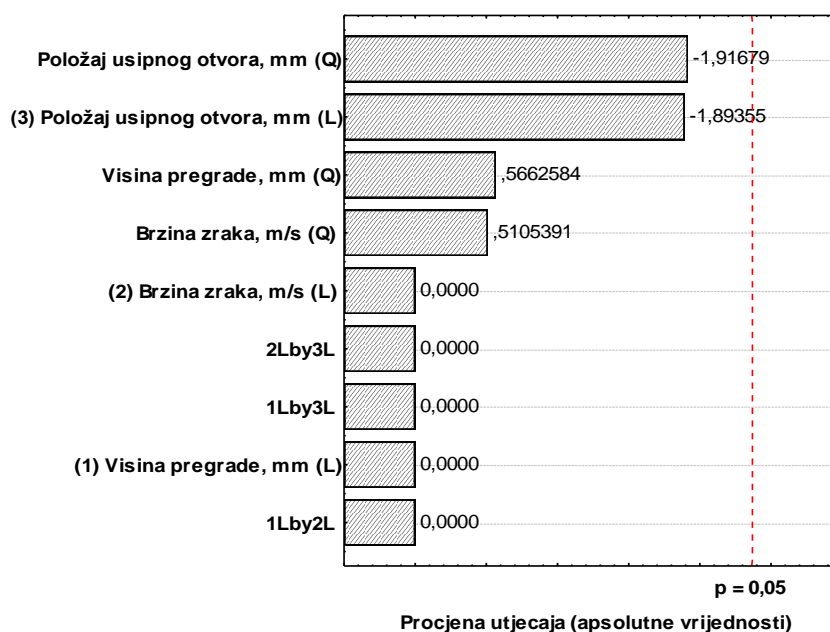
Grafikon 4 – 15 Procjena veličine utjecaja radnih parametara i njihovih međudjelovanja na kvalitetu koncentrata klase -0,5 mm – grupa „OSKKŽ“
