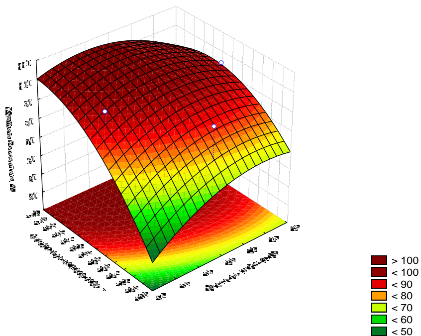
Slika 4 – 214 Regresijska ploha ovisnosti kvalitete koncentrata klase 2/1 mm o položaju separacijskog noža i napona na elektrodi – grupa „TP“
