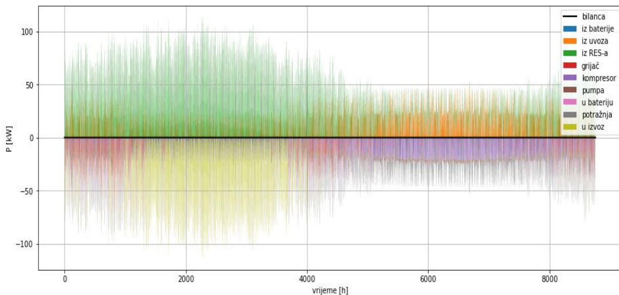
Slika 6-1. Energetske tokovi modela 27
